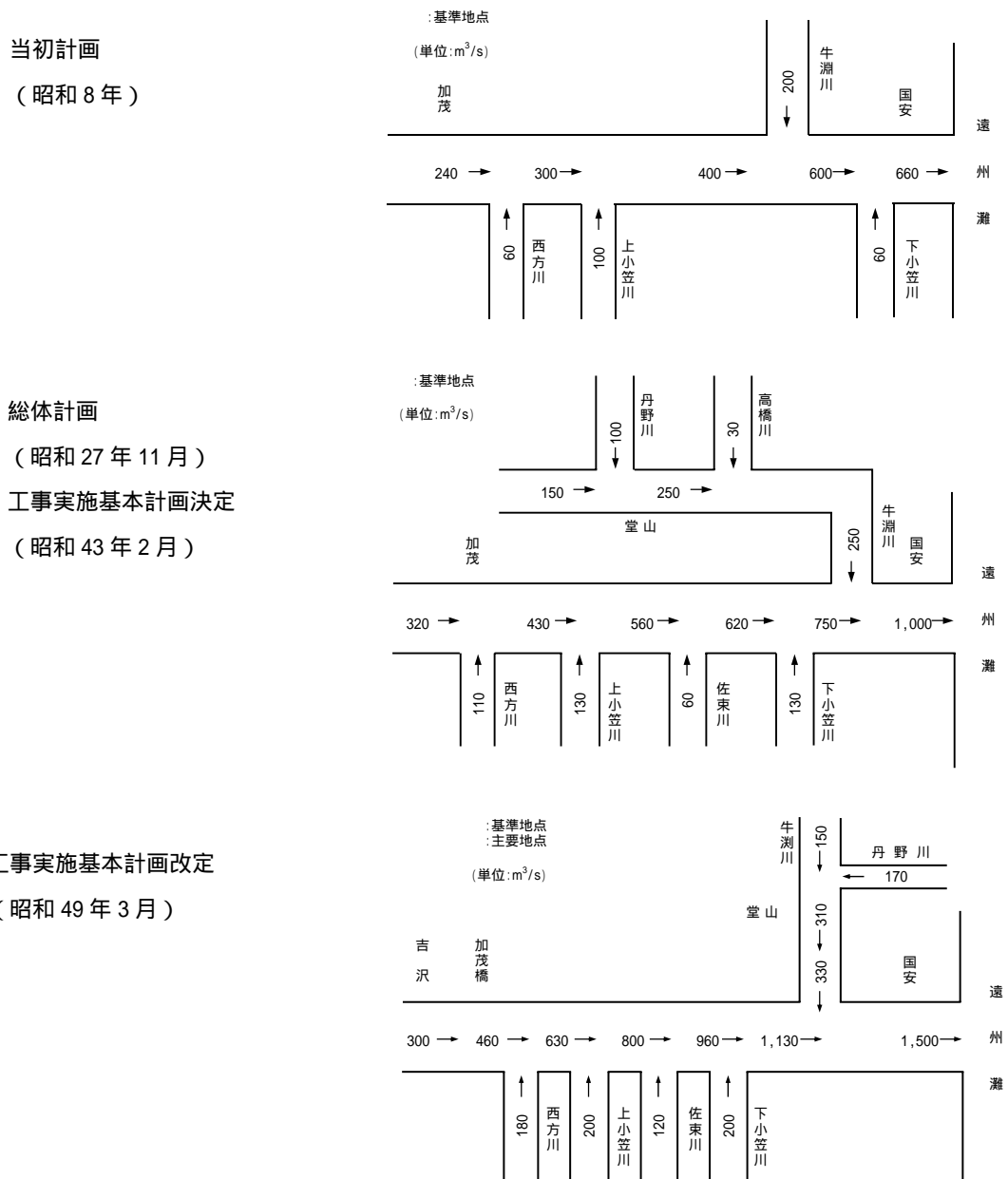
図-4.19 既定計画の変遷
