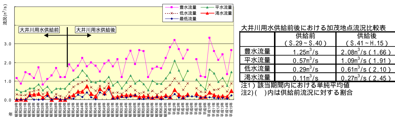
図-5.1 河川流況（加茂地点）
