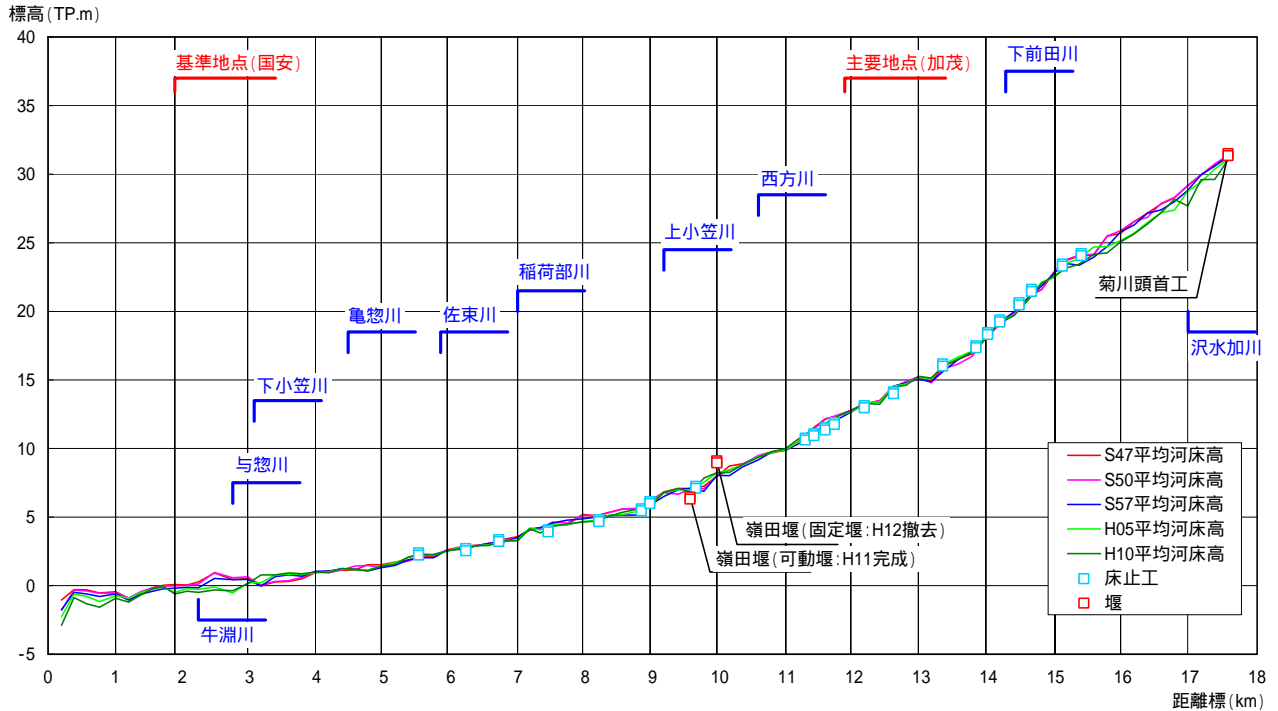
図-8.4 平均河床高縦断面図の経年変化
