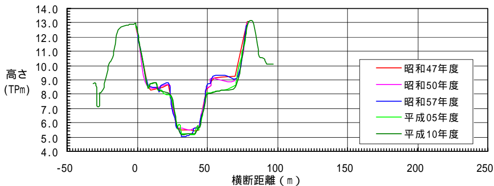
中流部（9.0k）の横断面図
