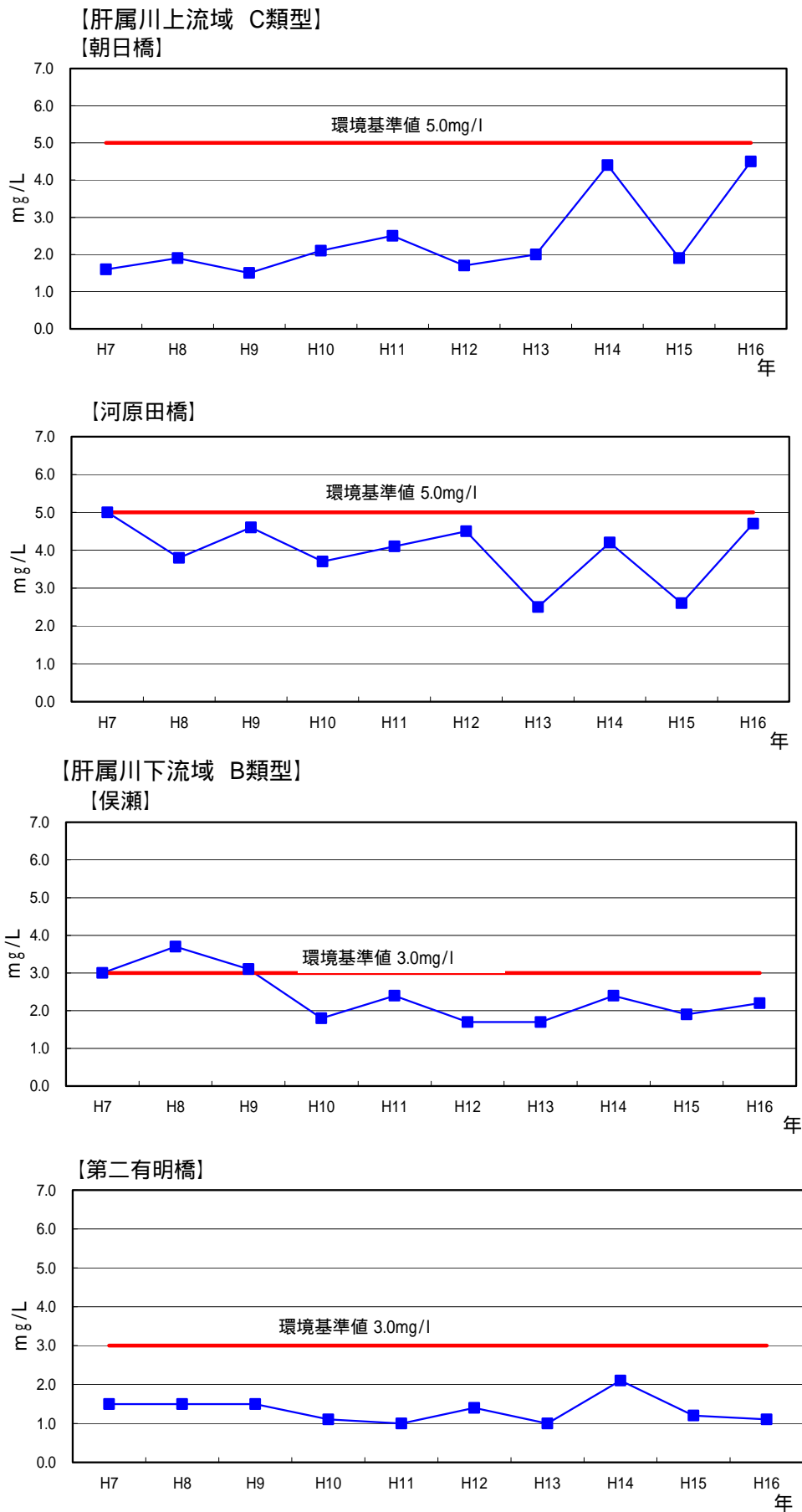
図 5-2 水質観測地点の BOD75% 値経年変化図
