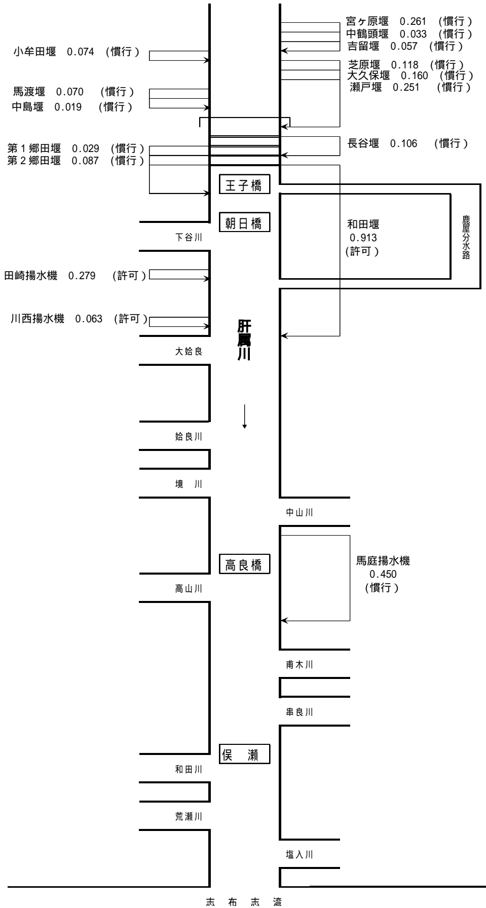
図 2-2 肝属川水系の主な水利用の現況模式図
