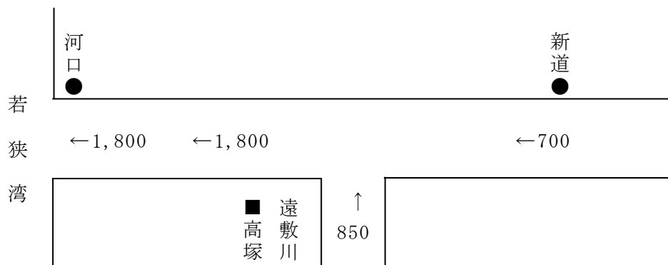
北川計画高水流量図 (単位： \text{m}^3/\text{s} )
