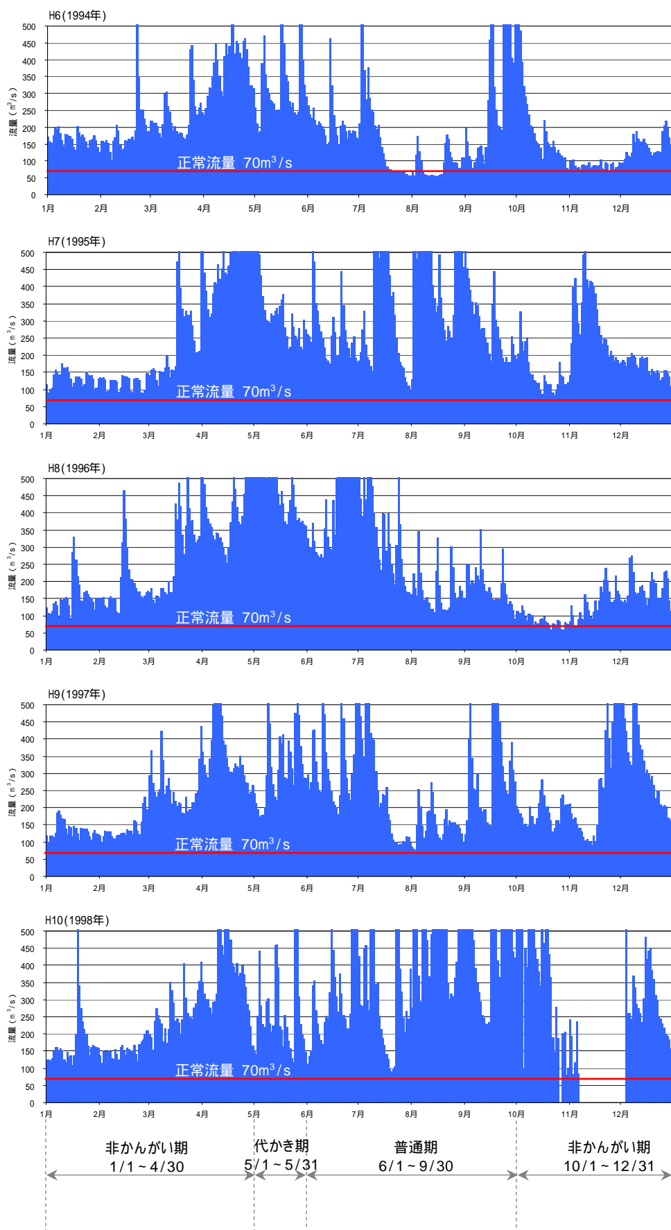
図 6-4(1) 日平均流量図 (狐禅寺地点: H6 ~ H10)
