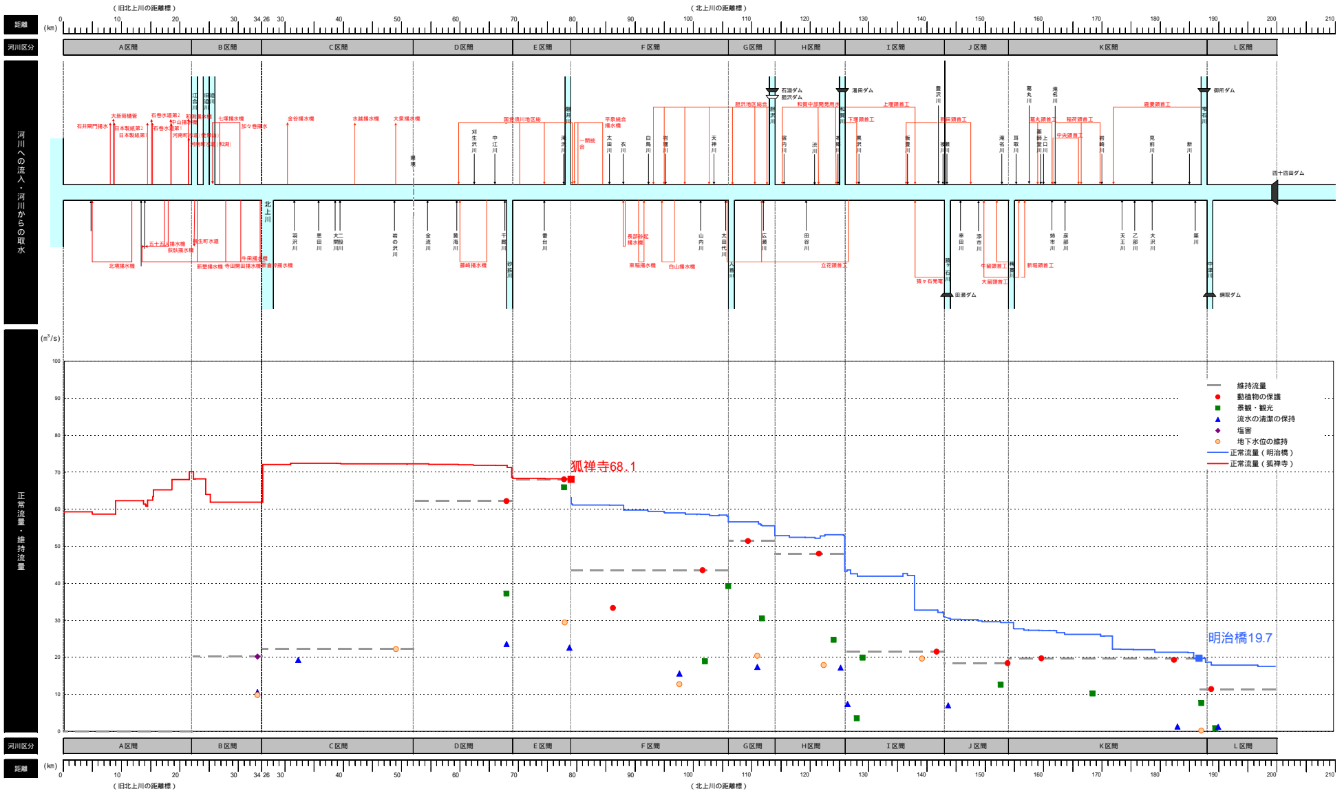
図 6-3 北上川正常流量図（非かんがい期 10～4月）
