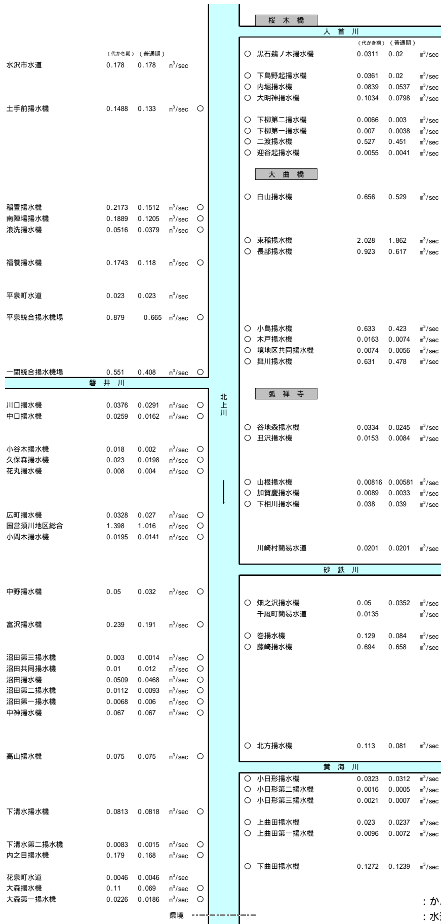
図 2-2(2) 北上川上流部 水利模式図
