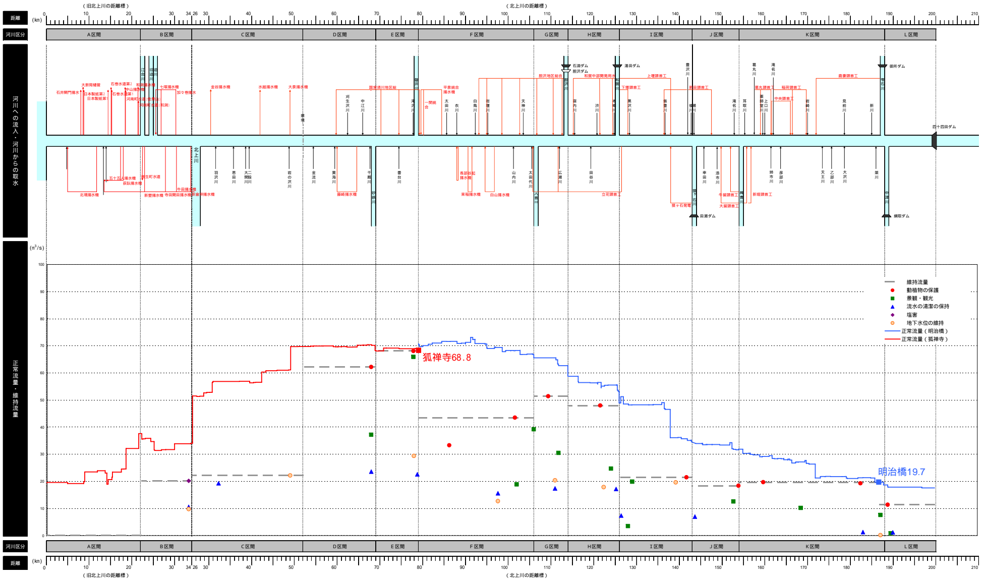
図 6-2 北上川正常流量図 (普通期 6~9月)
