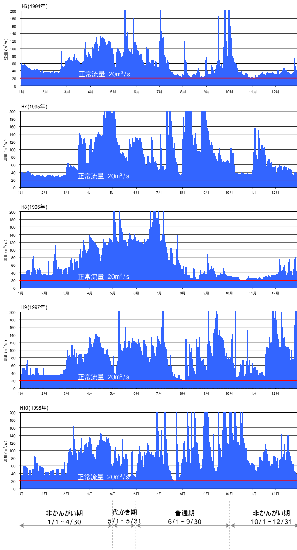
図 6-5(1) 日平均流量図 (明治橋地点: H6 ~ H10)
