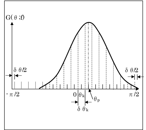
図4-19：波向の分割
