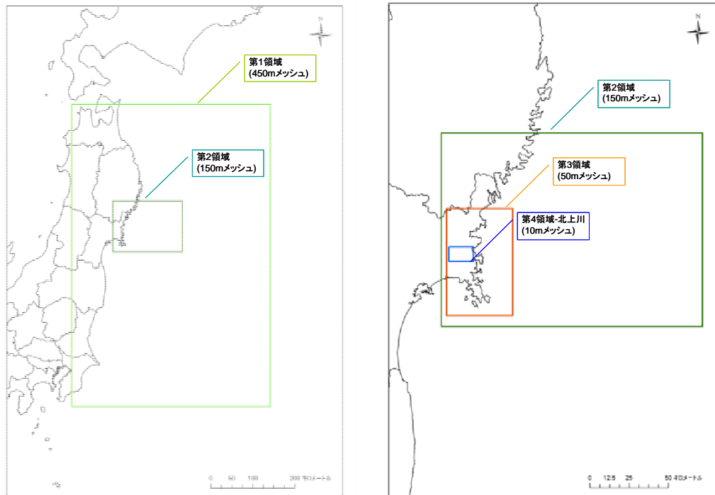
図 4-5：メッシュ接続位置図（北上川の例）
