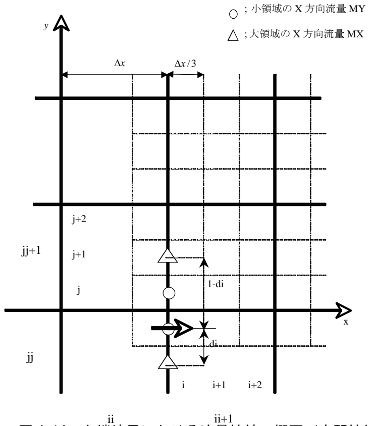
図 4-14 : 左端境界における流量接続の概要 (空間接続 1/3)
