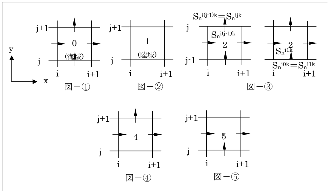
図 4-20 : 波向の分割
