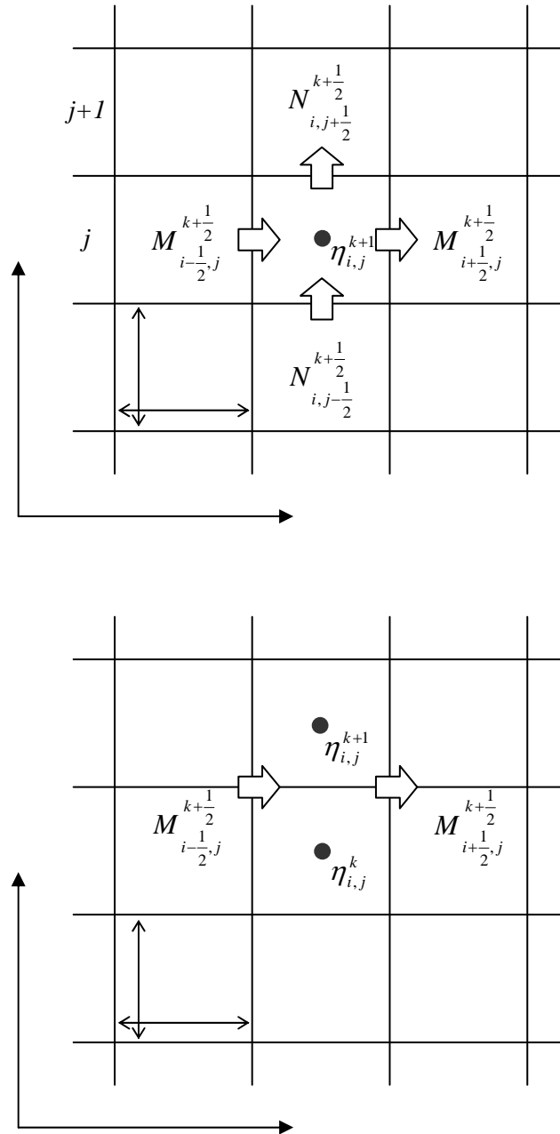
図 4-12 : Leap-frog 法の計算点の配置 (Staggered 格子)
