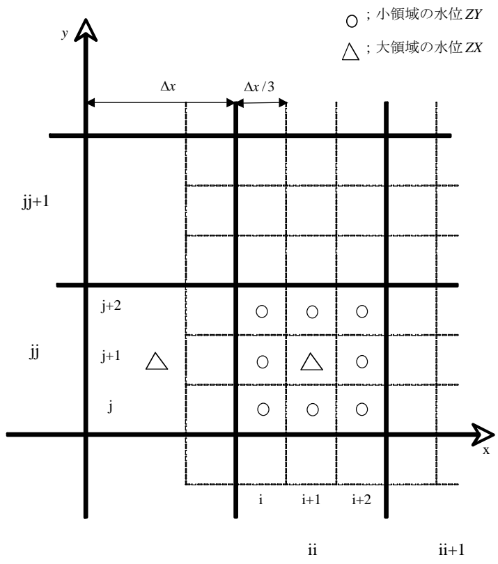
図 4-13 : 左端境界における水位接続の概要 (空間接続 1/3)
