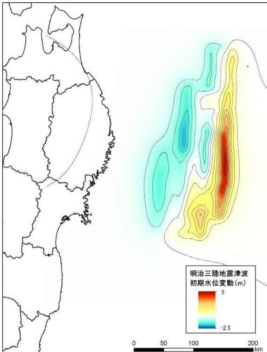
図 4-1 検討対象地震（明治三陸地震）での初期潮位変動量
