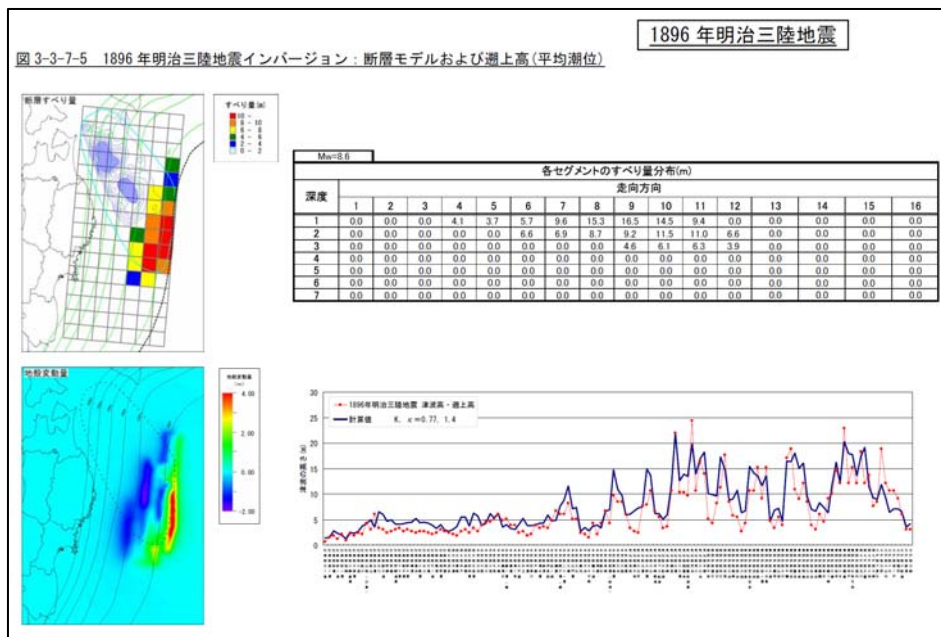
図 4-2：明治三陸地震の断層推定図
