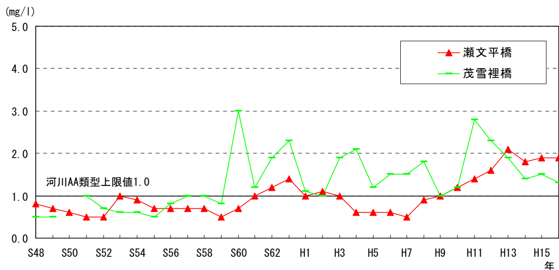
図 5-2 (1) 釧路川における水質 (BOD75%値) の経年変化 (AA 類型)
