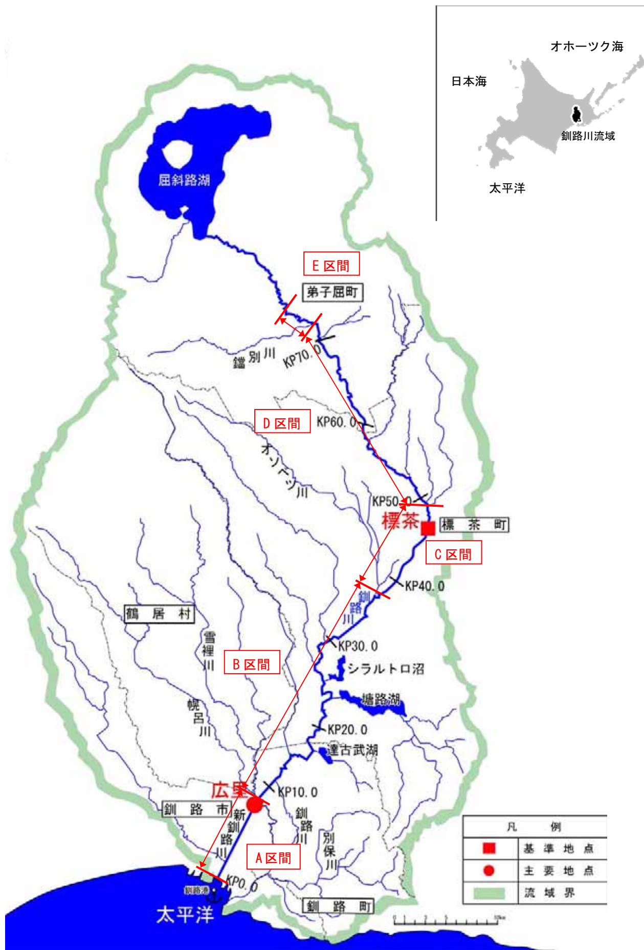
図 1-1 釧路川水系流域図
