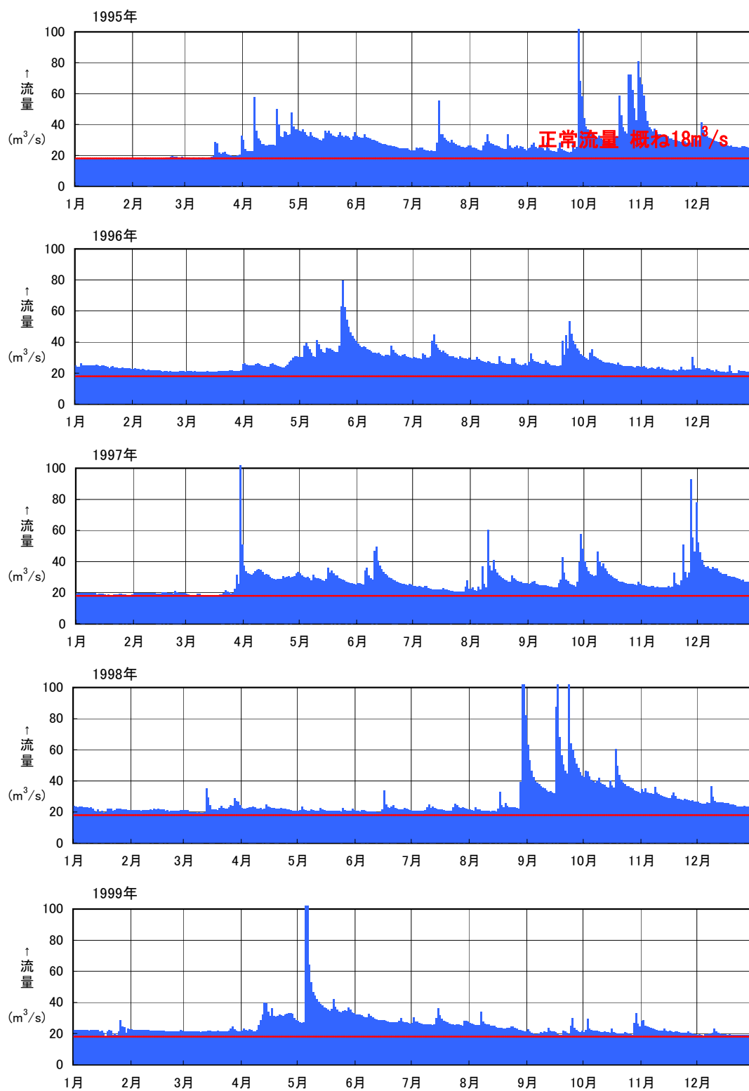
図 6-2 日平均流量図 (標茶地点 : 1995~1999年)
