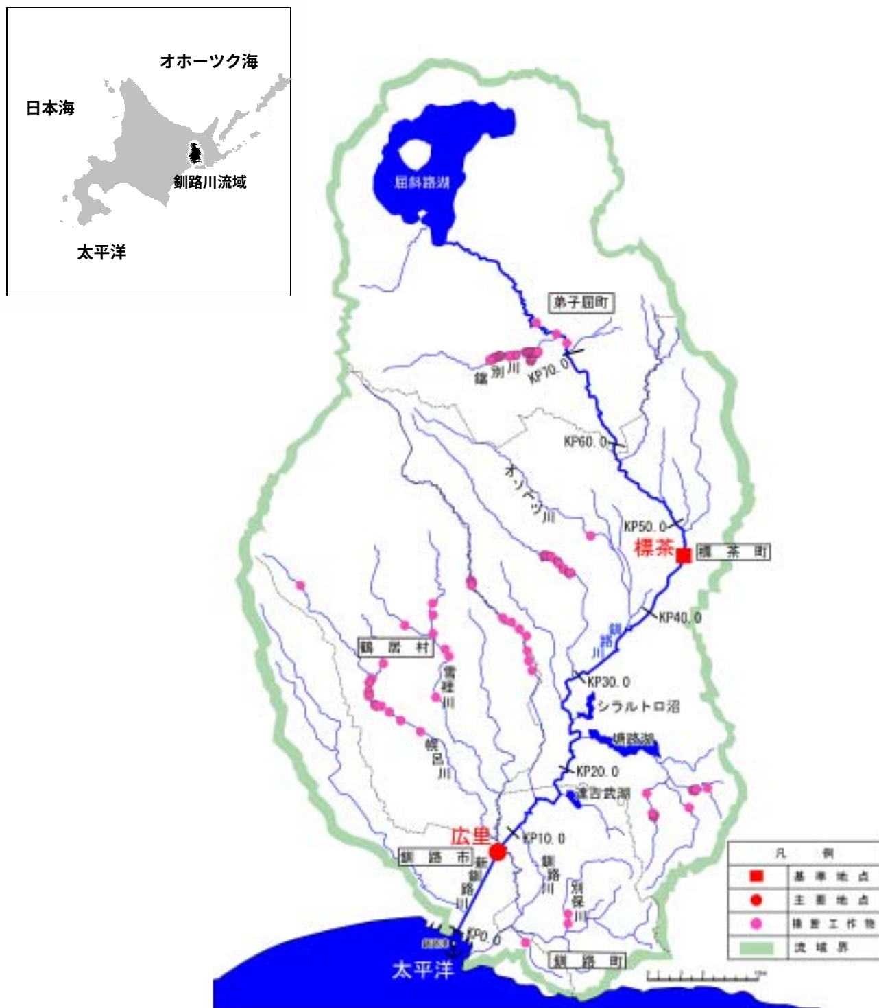
図 1-1 釧路川流域図
