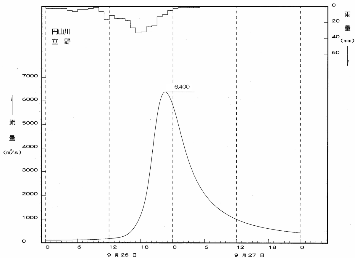
図 4-9 基本高水のハイドログラフ(立野地点、昭和 34 年 9 月型)
