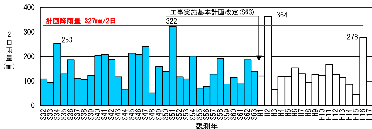
図 4-1 立野地点上流 年最大 2 日雨量
