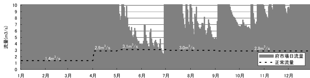
図 13 正常流量と日流量の比較(円山川府市場 H13~17)
