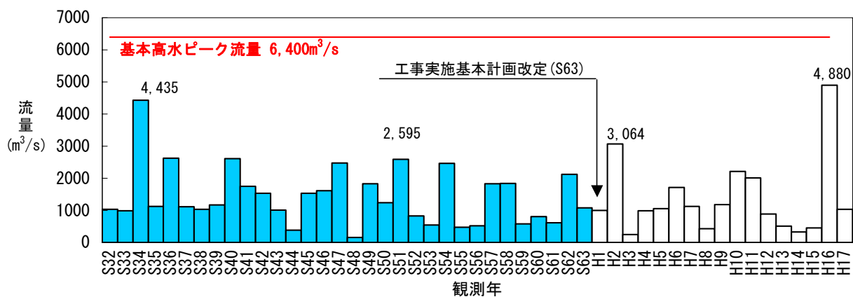
図 4-2 立野地点 年最大流量
