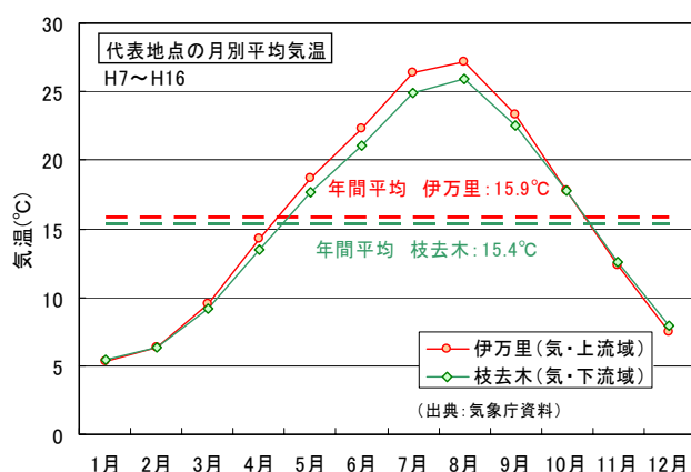
図 1- 5 代表地点の月別平均気温
