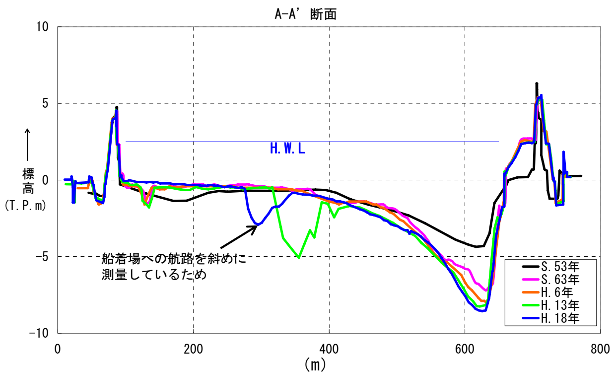
図 4-2 河口部横断変遷図
