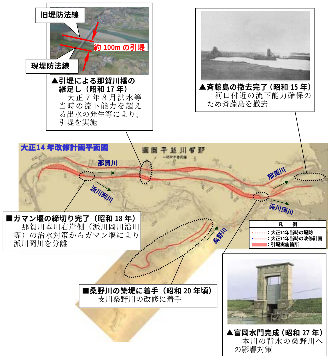
図4-4 那賀川的主要直轄改修事業
