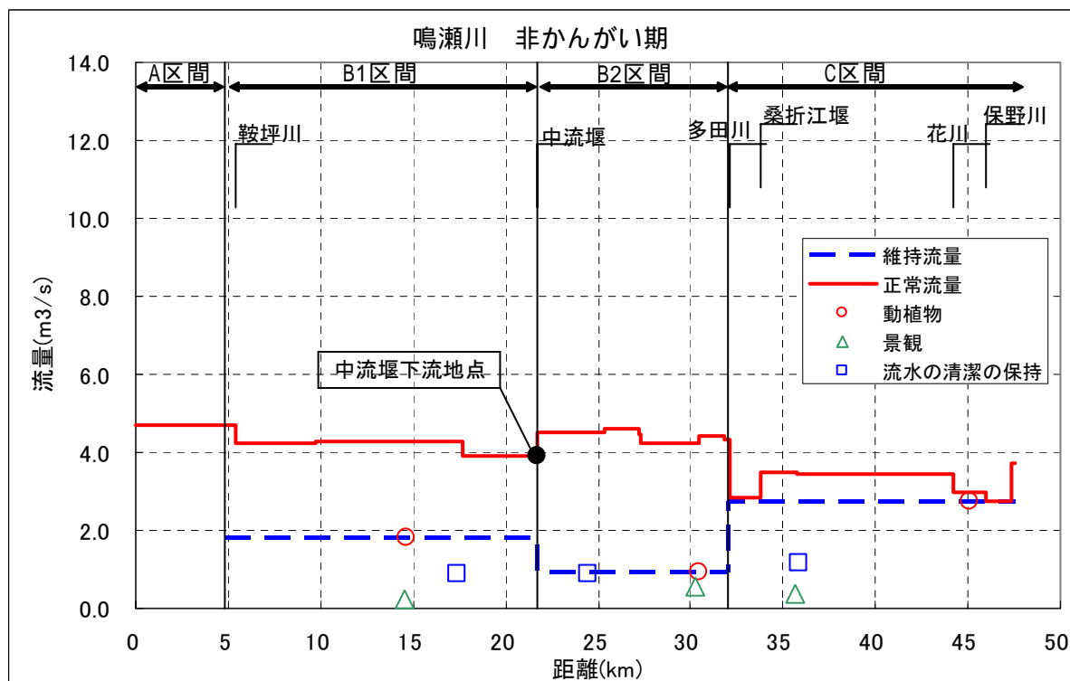
鳴瀬川正常流量縦断面図
