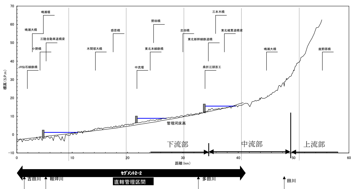
図 8-1 鳴瀬川河道縦断面図
