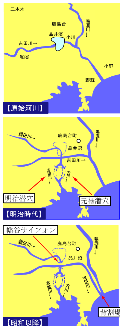
図 4-12 河道の変遷
