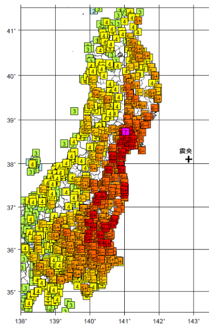
図 4-19 震度分布図
