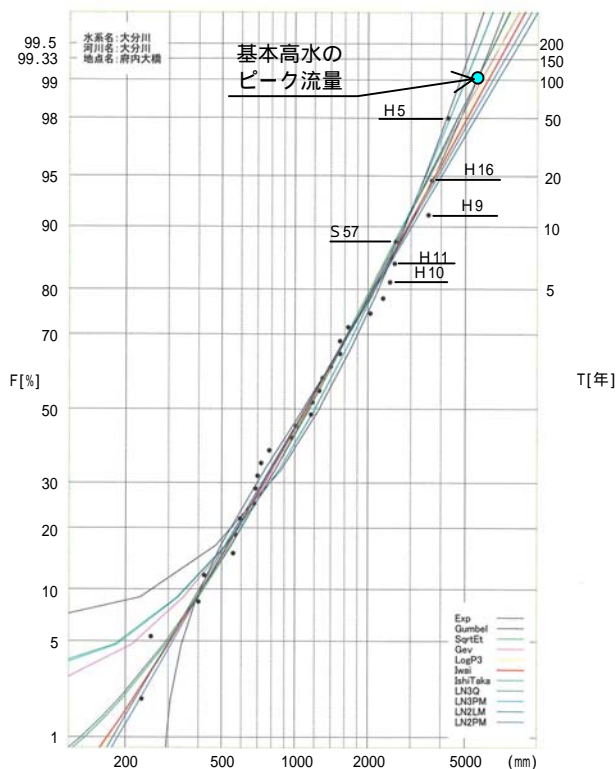
図4 - 7 府内大橋地点流量確率計算結果
