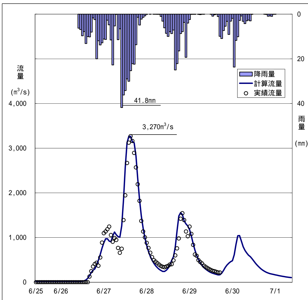
図4 - 2 昭和28年6月洪水再現計算結果(明礮橋地点)
