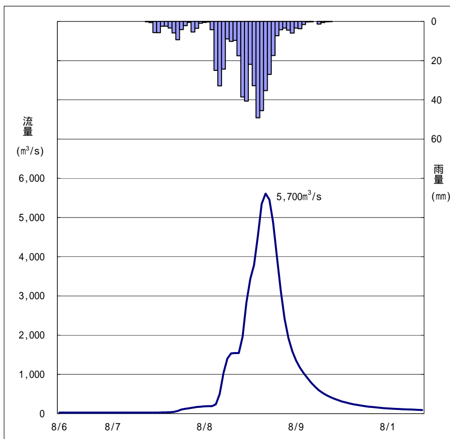
昭和34年8月型ハイドログラフ（府内大橋地点）
