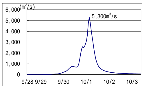
図 4 - 3 ハイドログラフの算定結果
