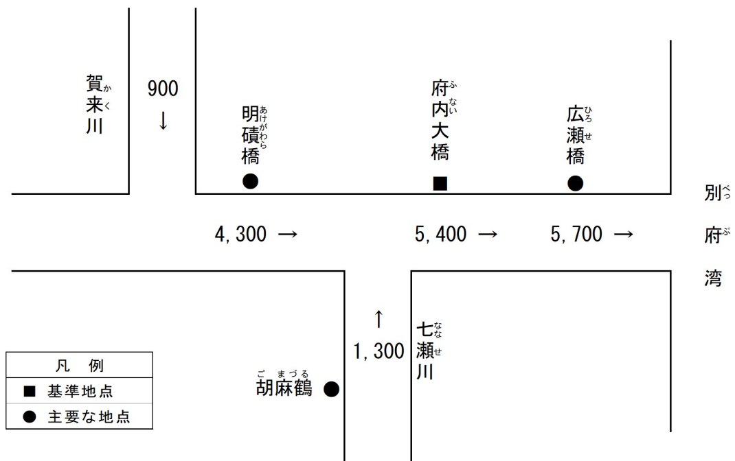
大分川計画高水流量図 (単位 : \text{m}^3/\text{s} )
