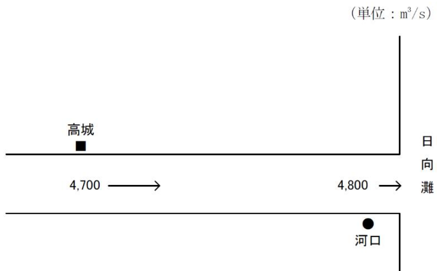
小丸川計画高水流量図
