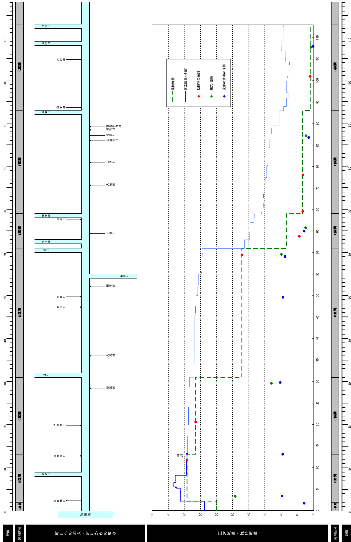
図 6-1 雄物川 正常流量縦断面図 (11~4月)
