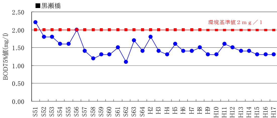
図 5-2 雄物川水系の水質経年変化図(BOD75%値)
