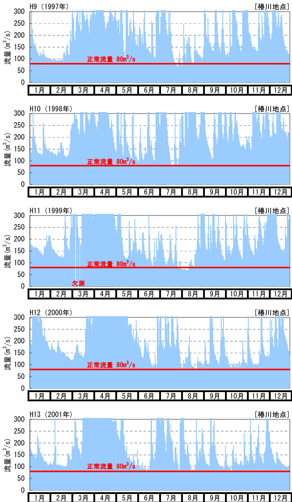
図 6-4(1) 日平均流量図(椿川地点 : H9~H13)
