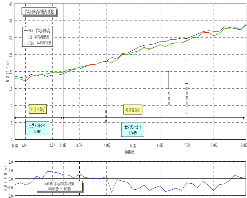
図 2-3 玉川平均河床高の経年変化
