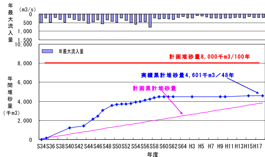
図 3-1 鎧畑ダム堆砂状況
