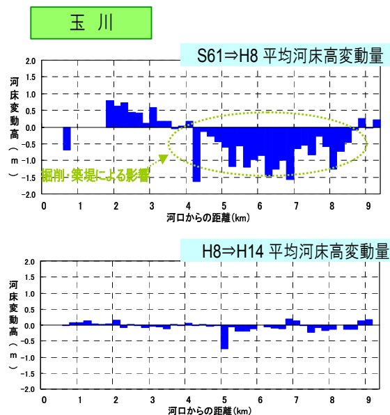
図 2-6 河床変動量の経年変化（玉川）
