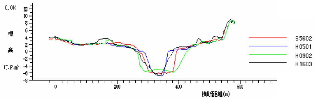
図 4-1 雄物川河口部 (0.0k) の横断面図
