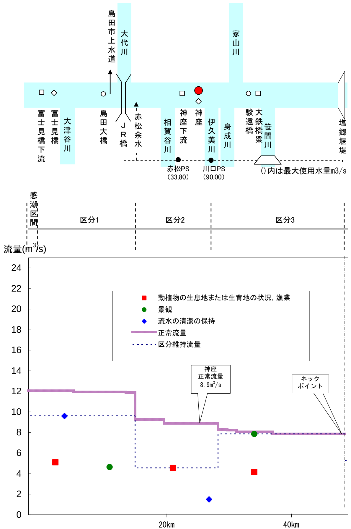
図 6.1 正常流量設定水収支縦断図（期間区分 1 1/1～2/28）
