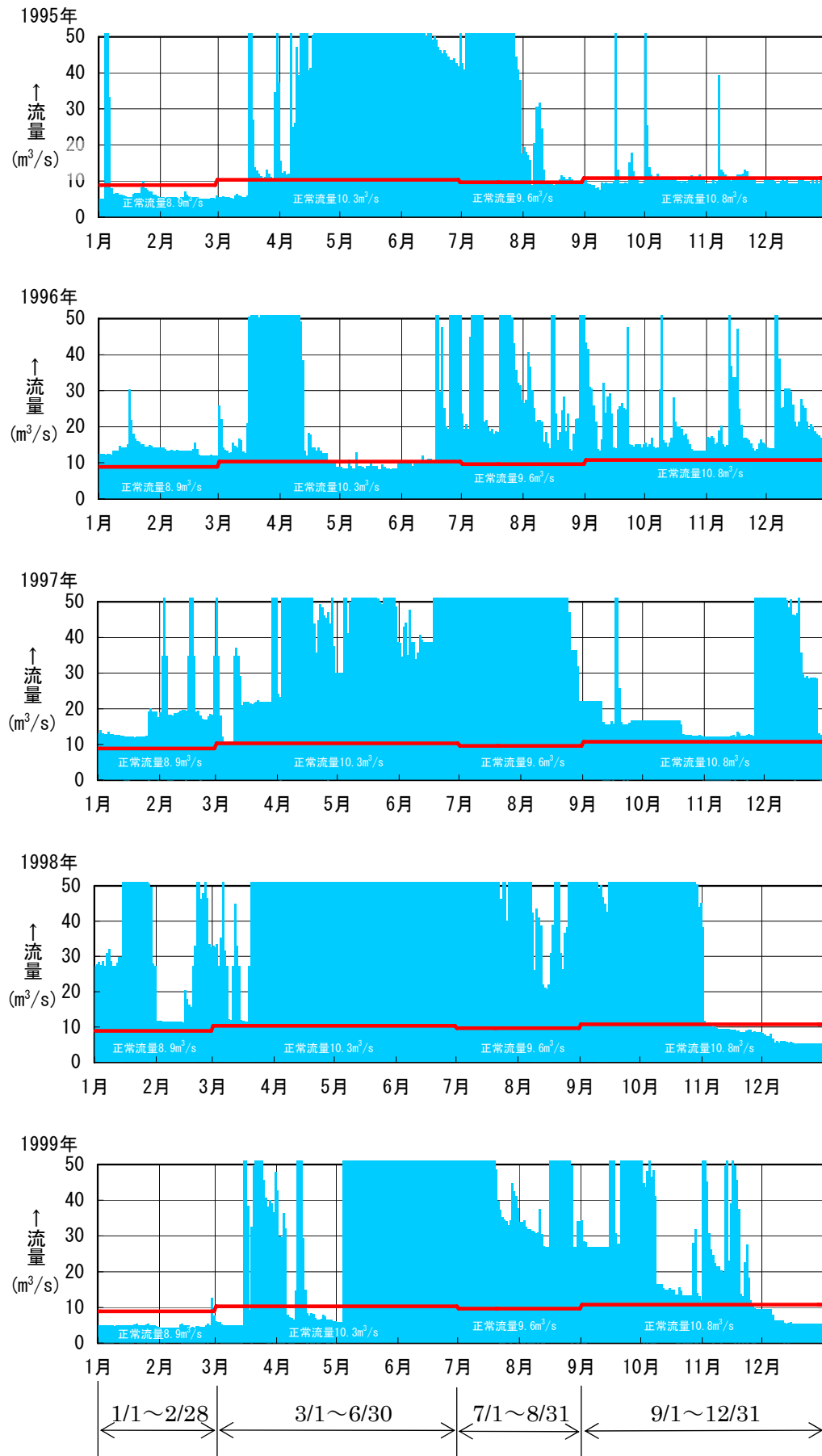
図 6.5 (1) 日平均流量図（神座地点：1995～1999 年）
