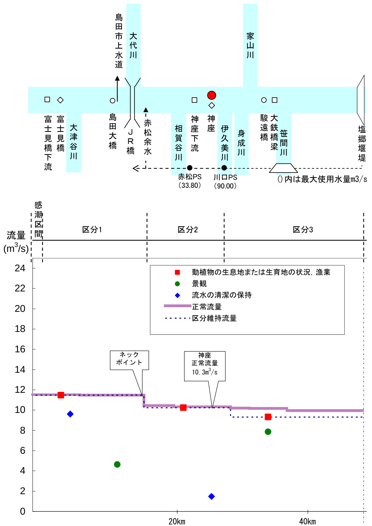
図 6.2 正常流量設定水収支縦断図（期間区分 2：3/1～6/30）
