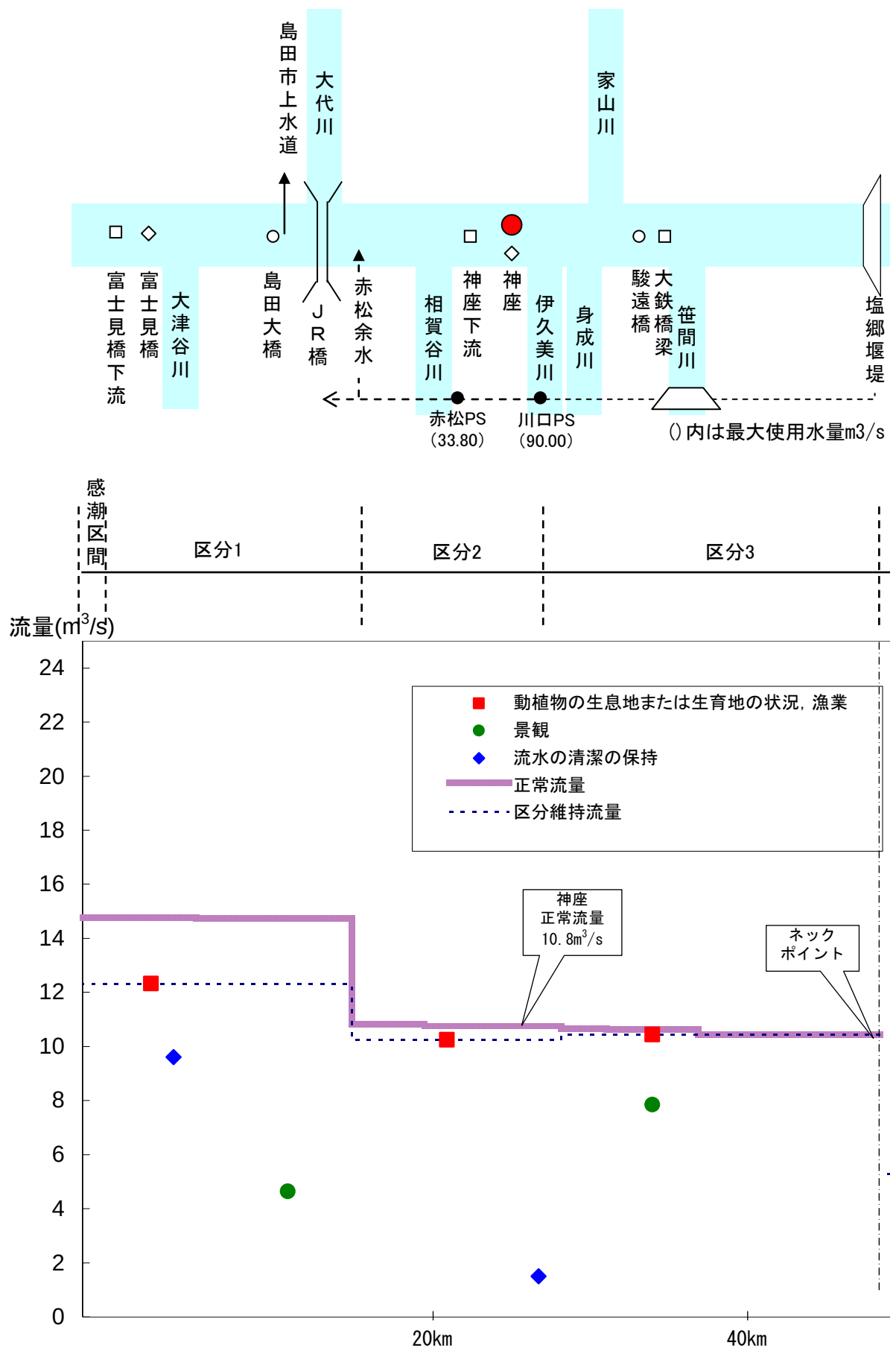
図 6.4 正常流量設定水収支縦断図 (期間区分 4 : 9/1~12/31)
