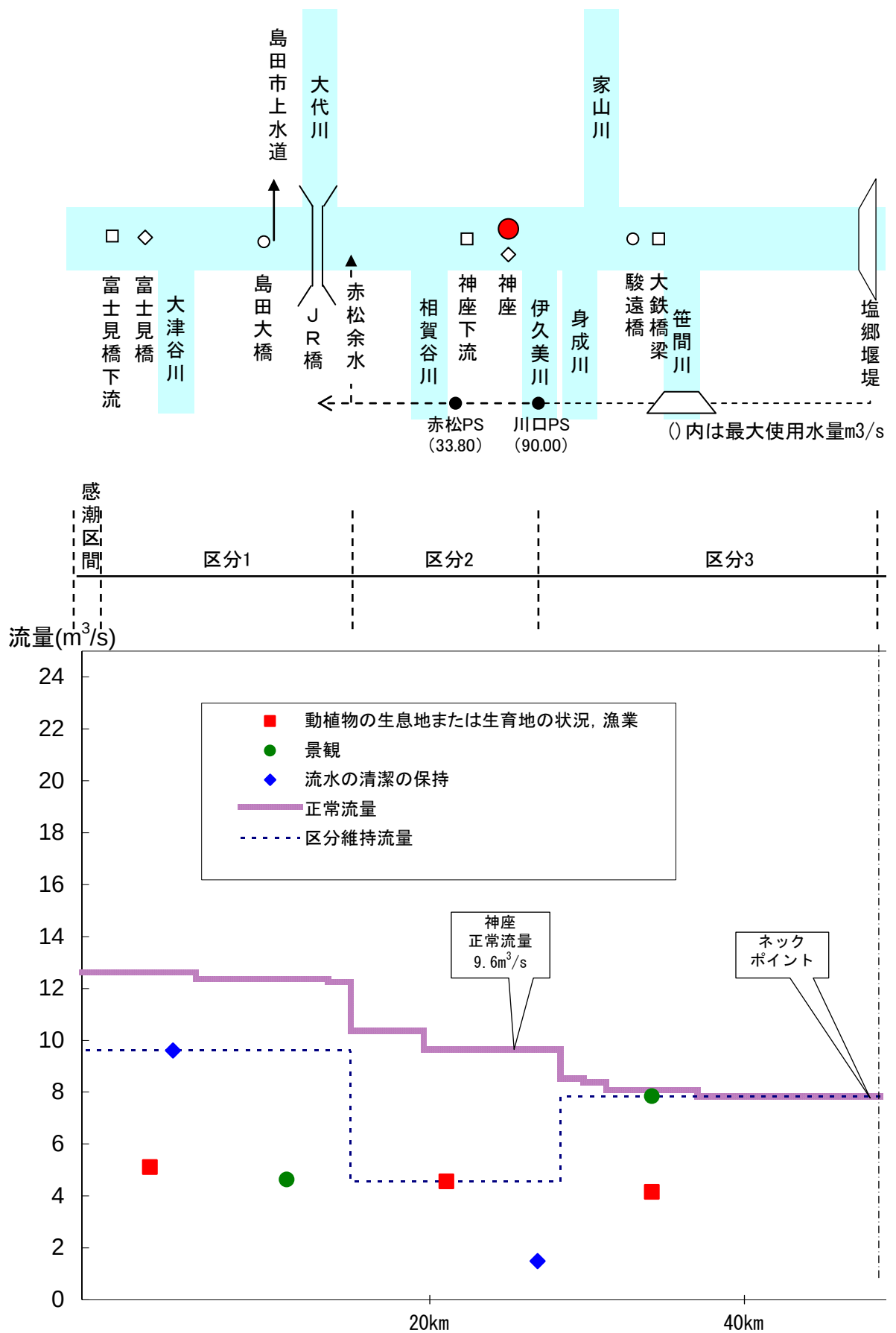
図 6.3 正常流量設定水収支縦断図（期間区分 3：7/1～8/31）
