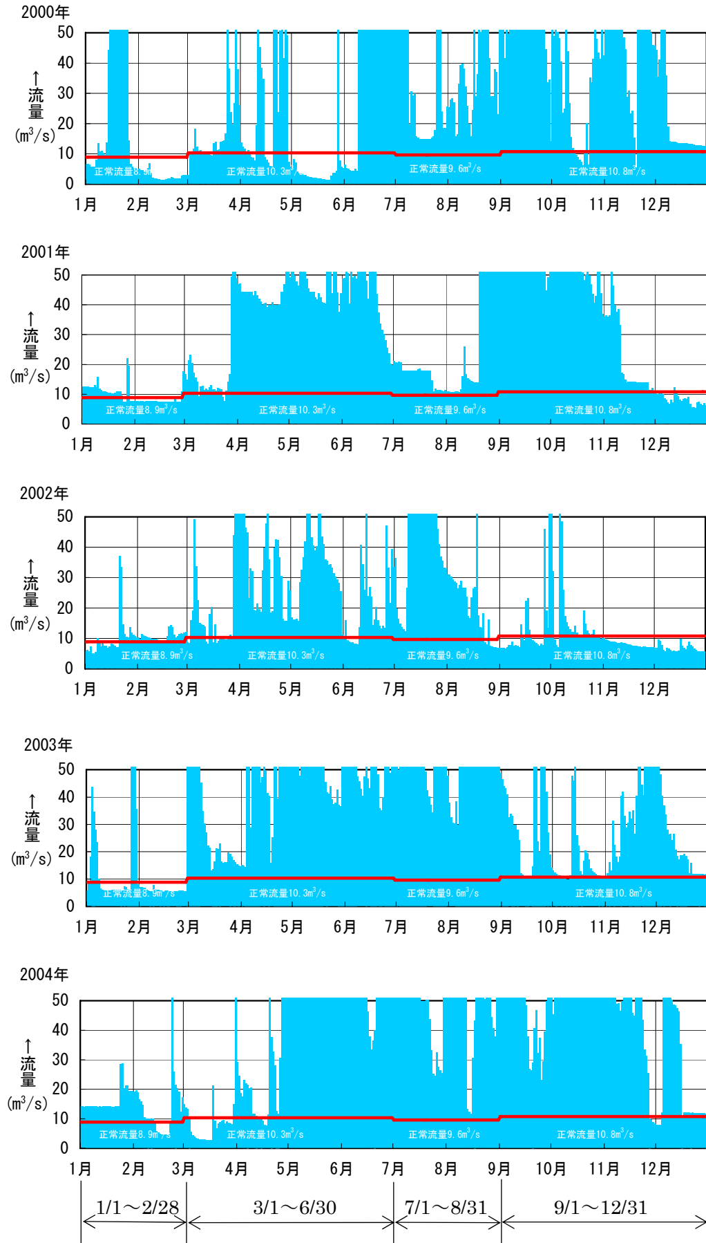
図 6.5 (2) 日平均流量図（神座地点：2000～2004 年）
