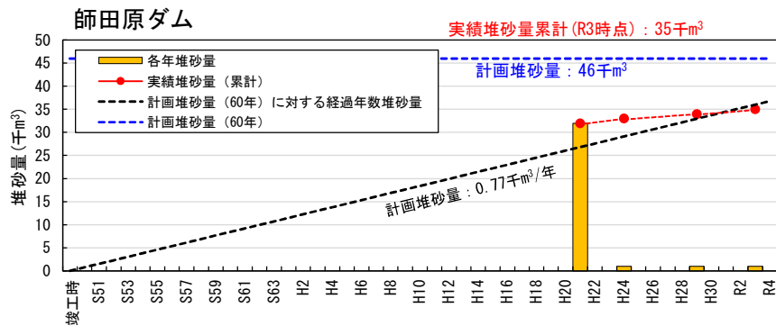
図 3.2(5) 師田原ダムの堆砂状況
