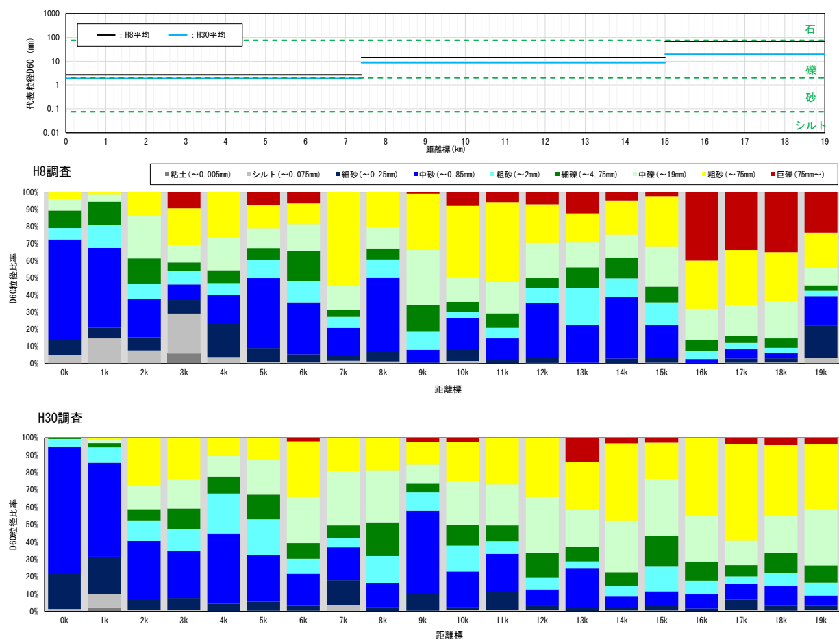
図 4.4(1) D60 粒径・粒径比率の縦断分布：大野川
