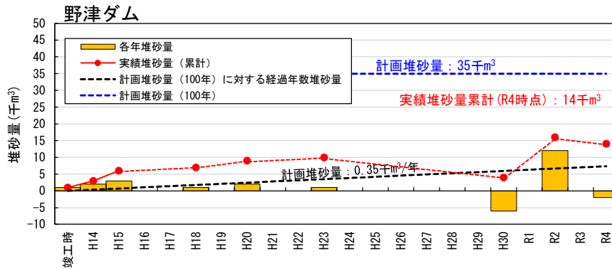
図 3.2(2) 野津ダムの堆砂状況
