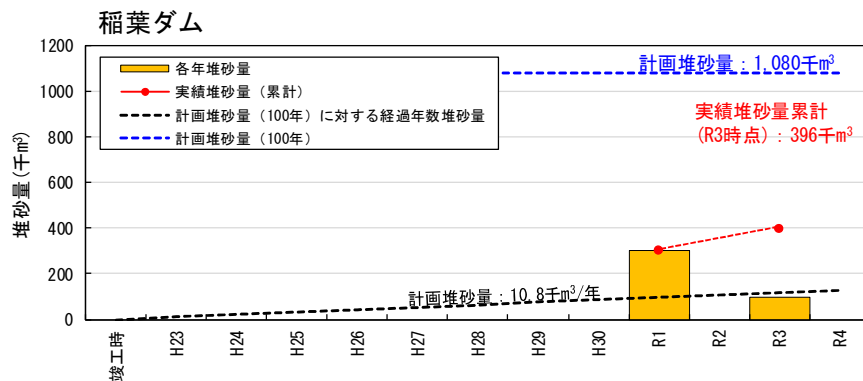
図 3.2(1) 稲葉ダムの堆砂状況
