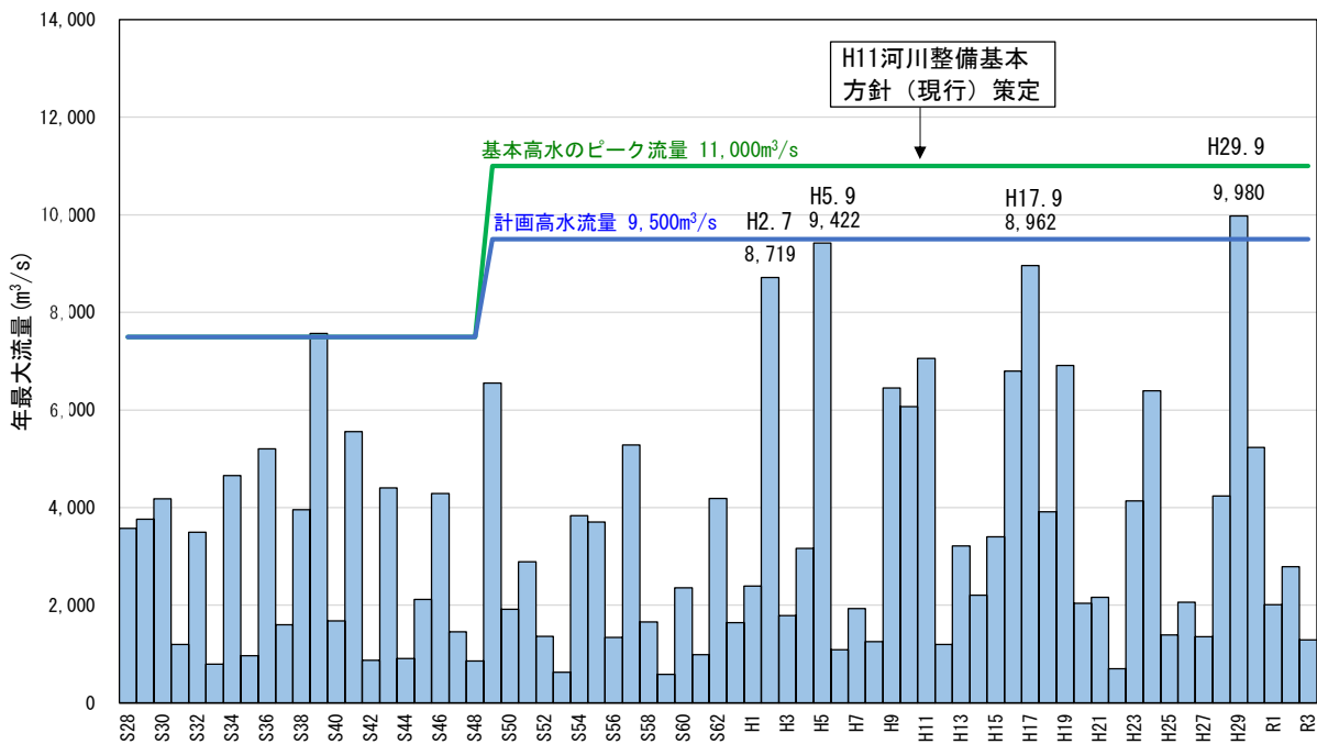
図 4.7 基準地点白滝橋における年最大流量の経年変化
