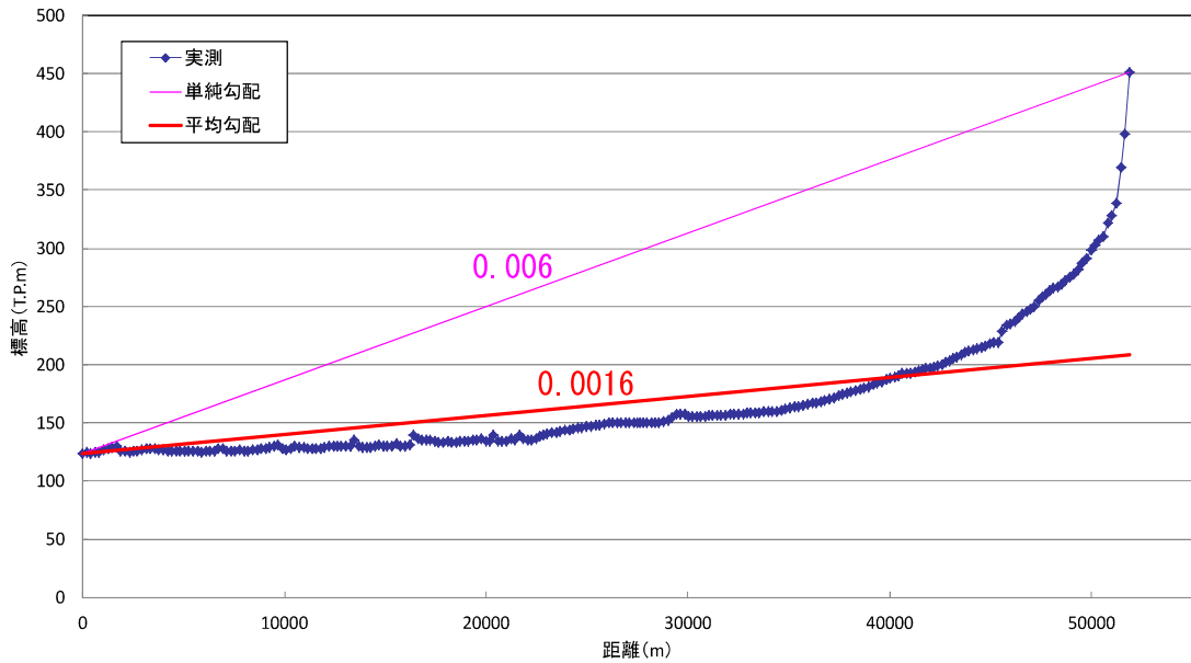
図 5. 4. 12 (2) 流路勾配、流路延長設定結果例（流域 1～樋渡地点）
