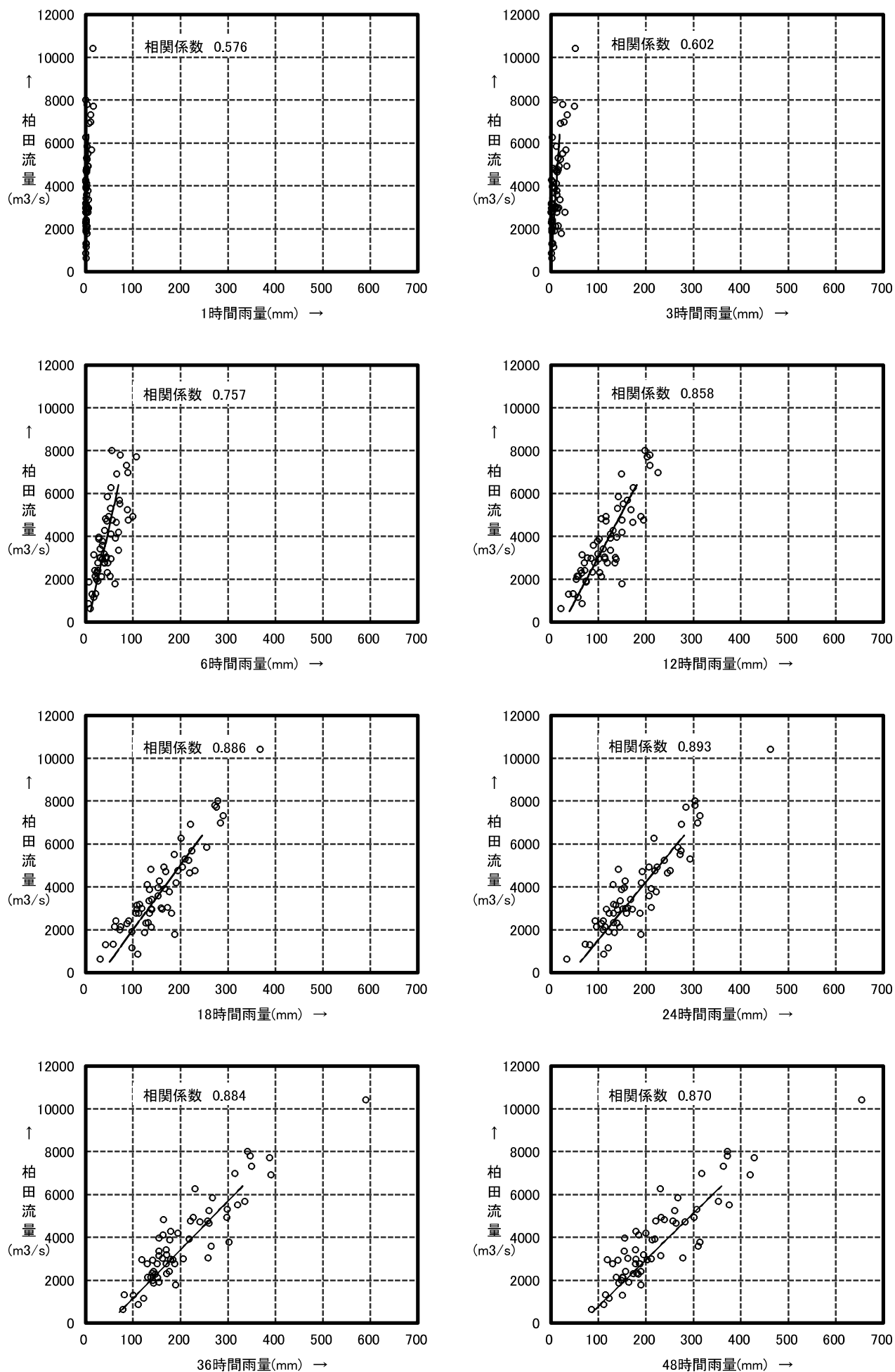
図6.3.4 ピーク流量と流域平均時間雨量の相関図
