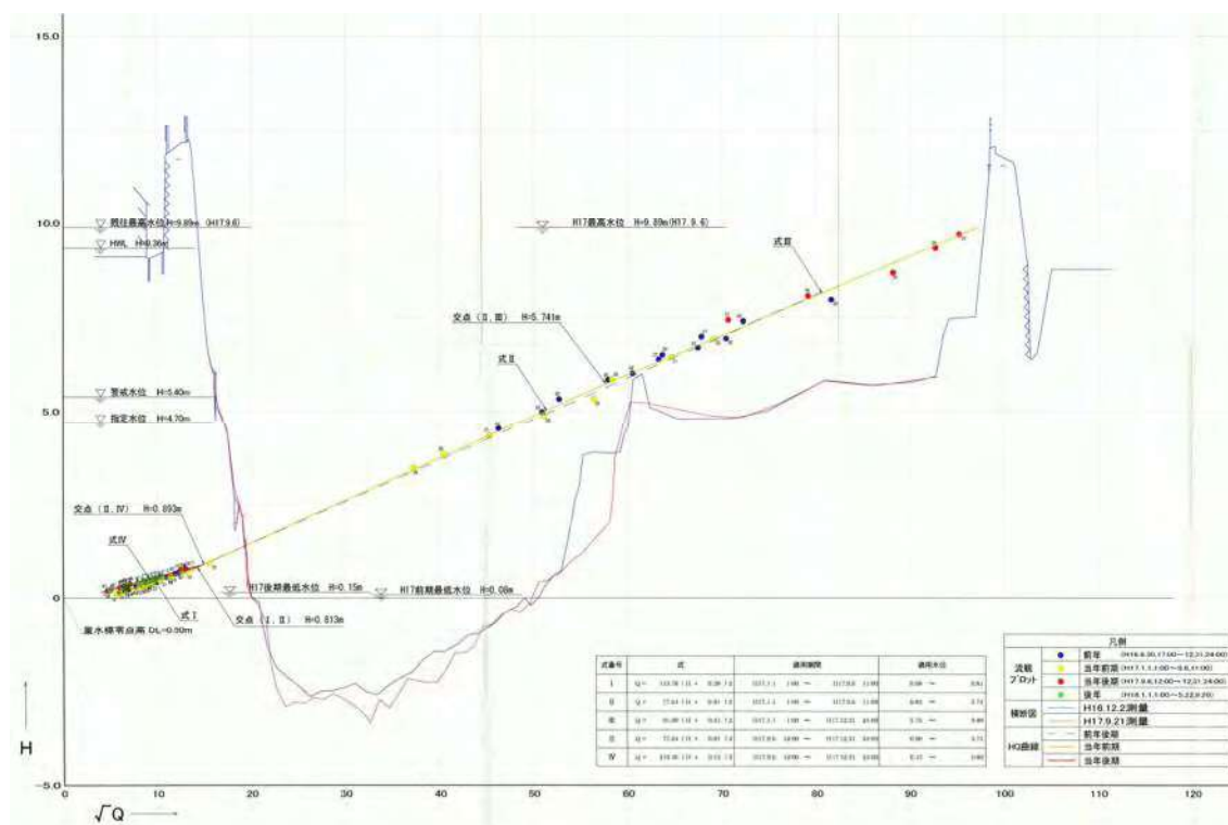
図 2.1.1 柏田地点における H \sim \sqrt{Q} 図 (平成 17 年 9 月出水)
