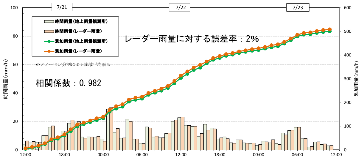
図 3.1.1 (3) 嵐田地点上流域における降雨ハイエトグラフ (H18.7 洪水)
