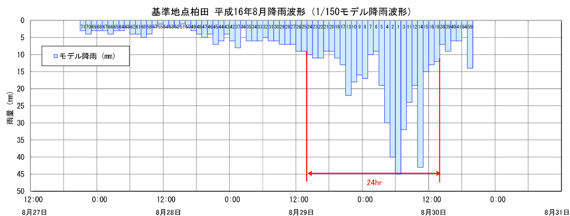
図 6. 9. 2(15) 1/150 モデル降雨波形における降雨ハイトグラフ (H16. 8)
