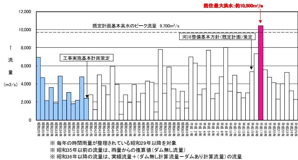
図 1.2.1 年最大流量 (基準地点柏田)
