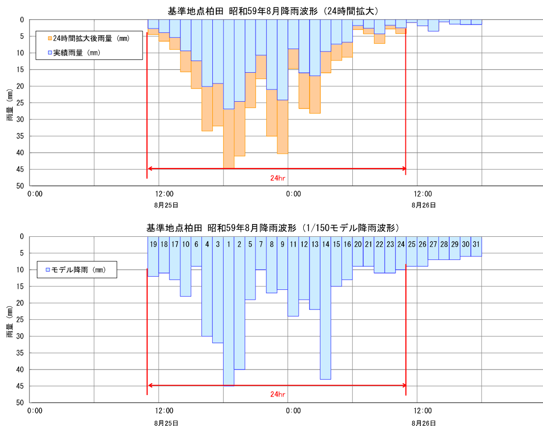
図 6.9.2(8) 1/150 モデル降雨波形における降雨ハイトグラフ (S59.8)
