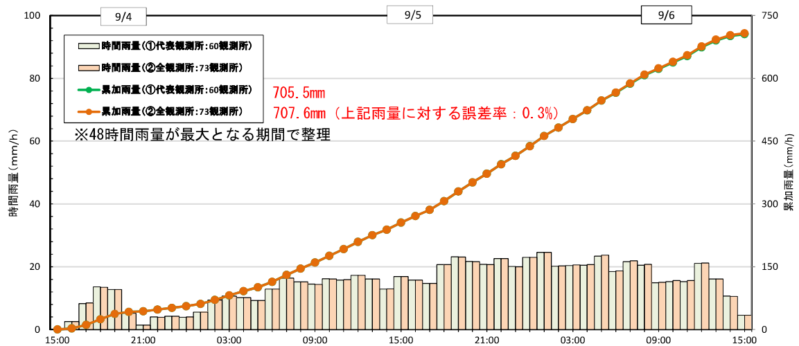
図 4. 2. 1 (1) 使用観測所数の違いによる流域平均雨量の比較 (柏田上流、H17.9 洪水)
