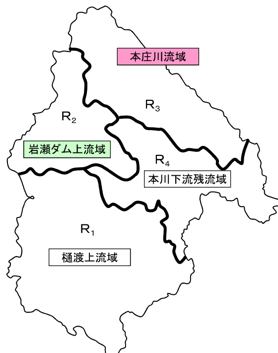
図 1.3.2 流域模式図
