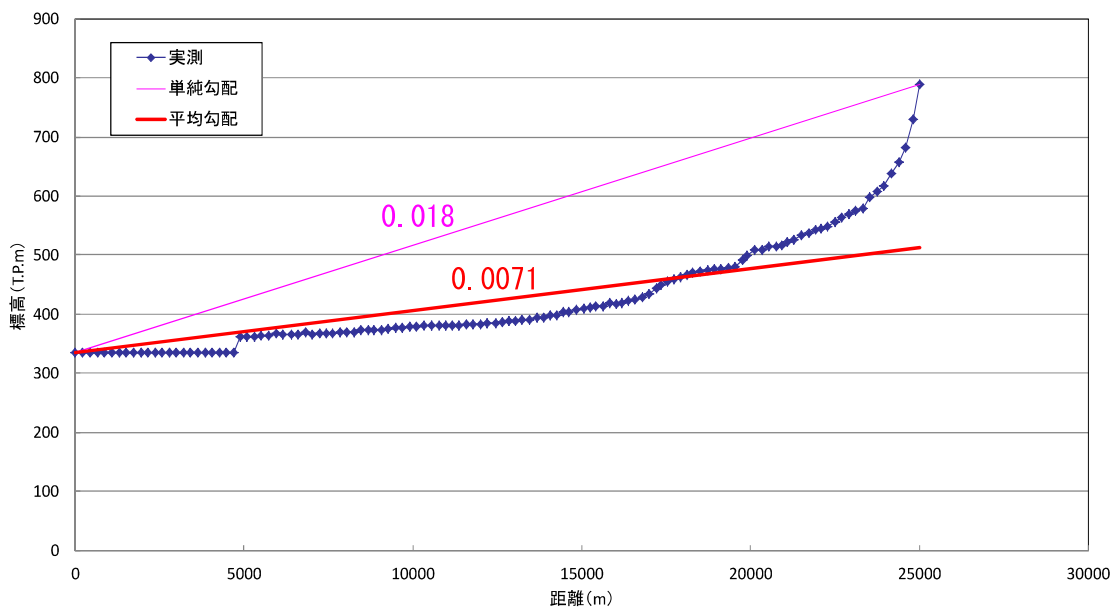
図 5. 4. 12 (4) 流路勾配、流路延長設定結果例（流域 43～綾南ダム地点）
