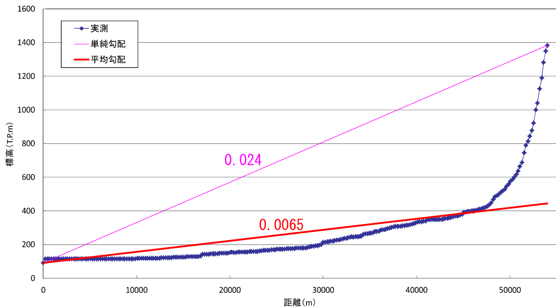
図 5. 4. 12 (3) 流路勾配、流路延長設定結果例（流域 25～岩瀬ダム地点）
