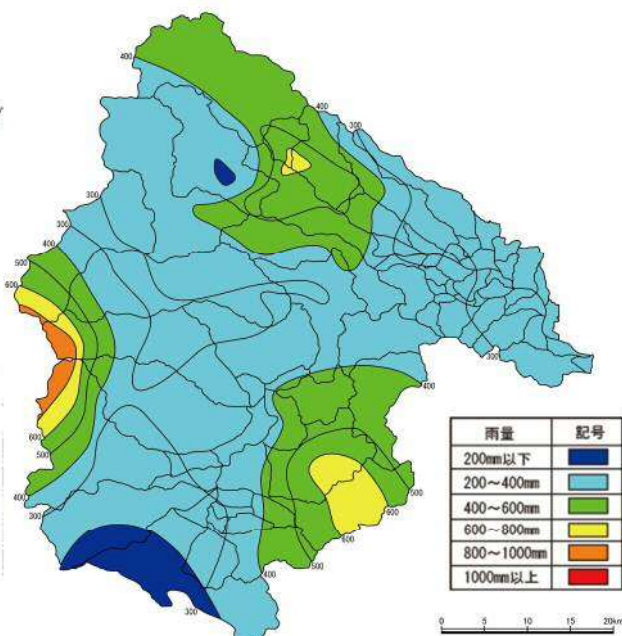
図 1.3.3(8) 台風経路図及び等雨量線図（平成9年9月16～17日洪水）
