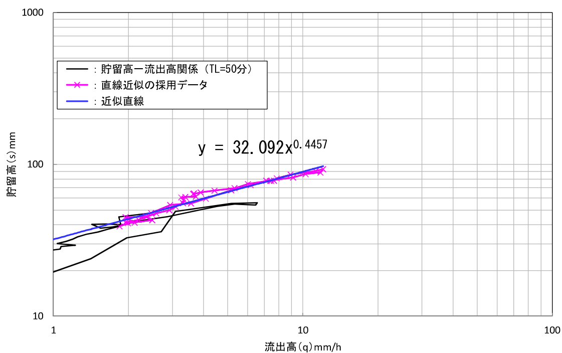
図5.4.8(3) 貯留高一流出高関係図(岩瀬ダム地点 H5.8.1洪水)
