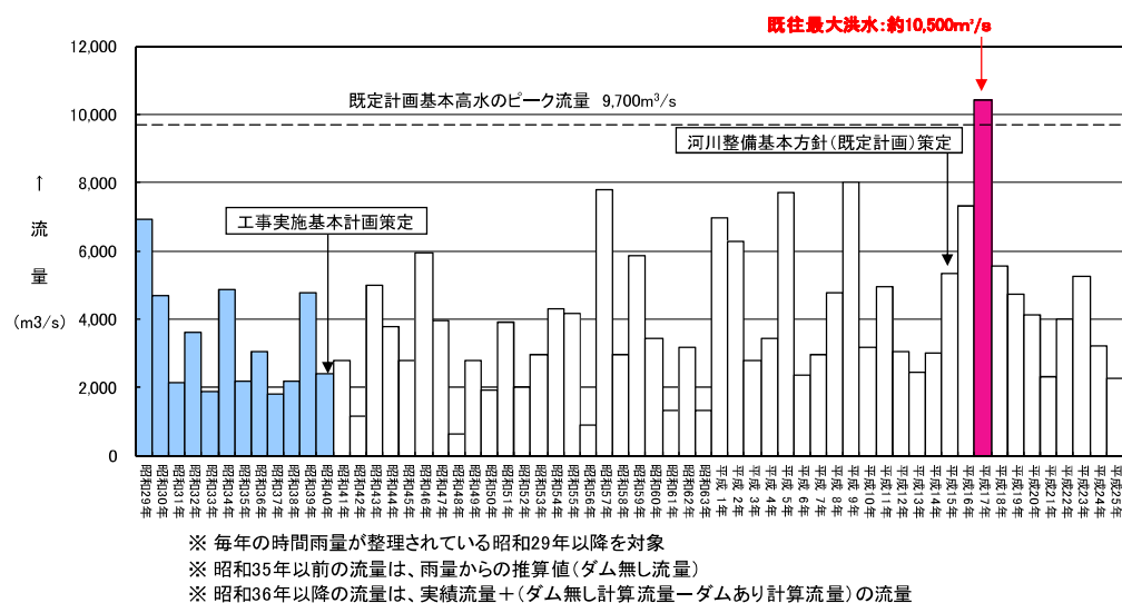
図 6.4.1 年最大流量（基準地点柏田）
