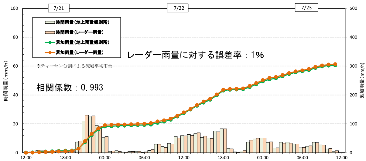
図 3.1.1 (2) 槇渡地点上流域における降雨ハイエトグラフ (H18.7 洪水)
