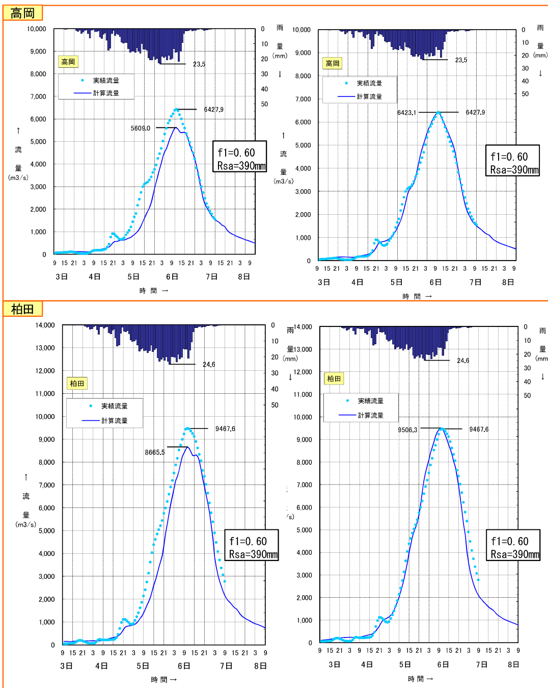
図 1(2) 平成 17 年 9 月洪水の再現性の比較
