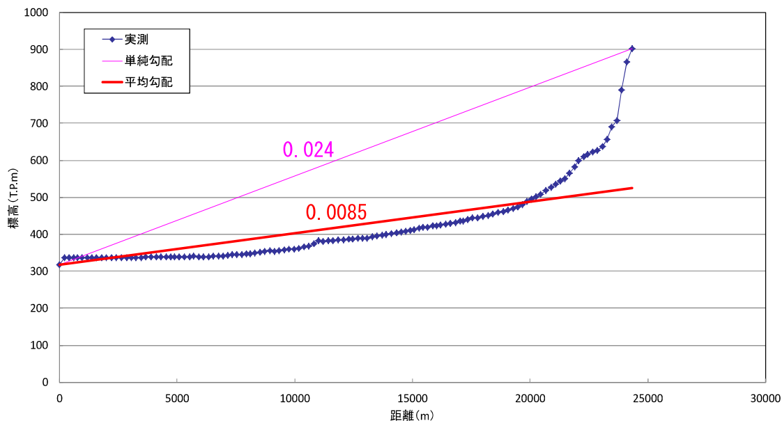
図 5. 4. 12 (5) 流路勾配、流路延長設定結果例（流域 47～田代八重ダム地点）
