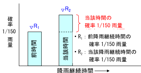
図 6.9.1 モデル降雨波形の作成方法
