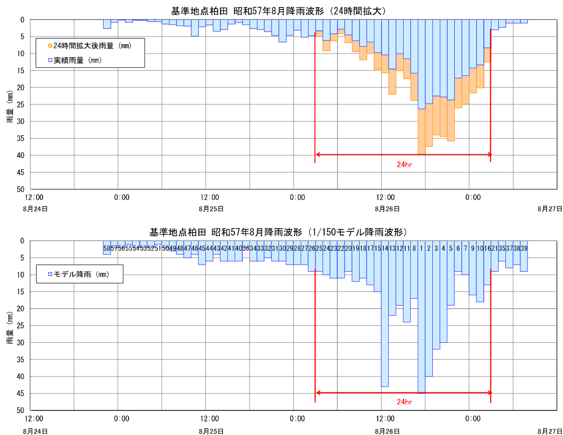
図 6.9.2(7) 1/150 モデル降雨波形における降雨ハイトグラフ (S57.8)
