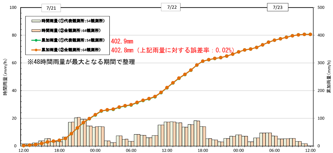
図 4. 2. 1 (2) 使用観測所数の違いによる流域平均雨量の比較 (柏田上流、H18.7 洪水)
