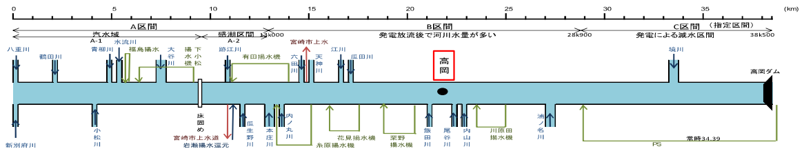
大淀川下流 正常流量 水収支縦断面図(非かんがい期:10/11~11/30,3/1~6/10)
