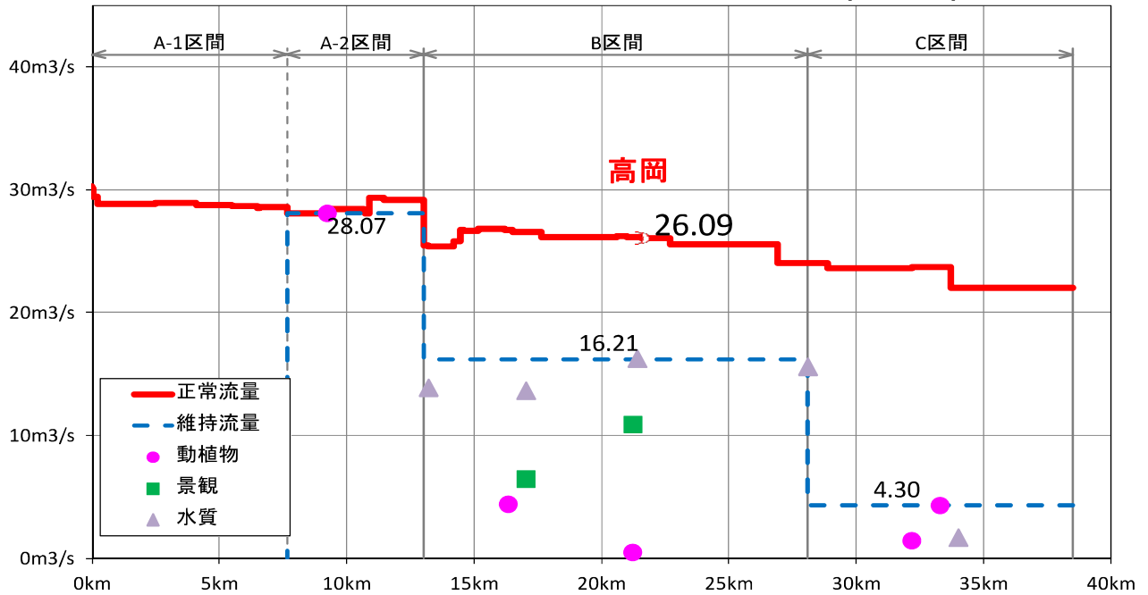
大淀川下流 正常流量 水収支縦断面図(かんがい期:6/11~10/10)
