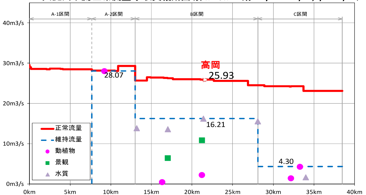
大淀川下流 正常流量 水収支縦断面図(非かんがい期:10/11~11/30,3/1~6/10)
