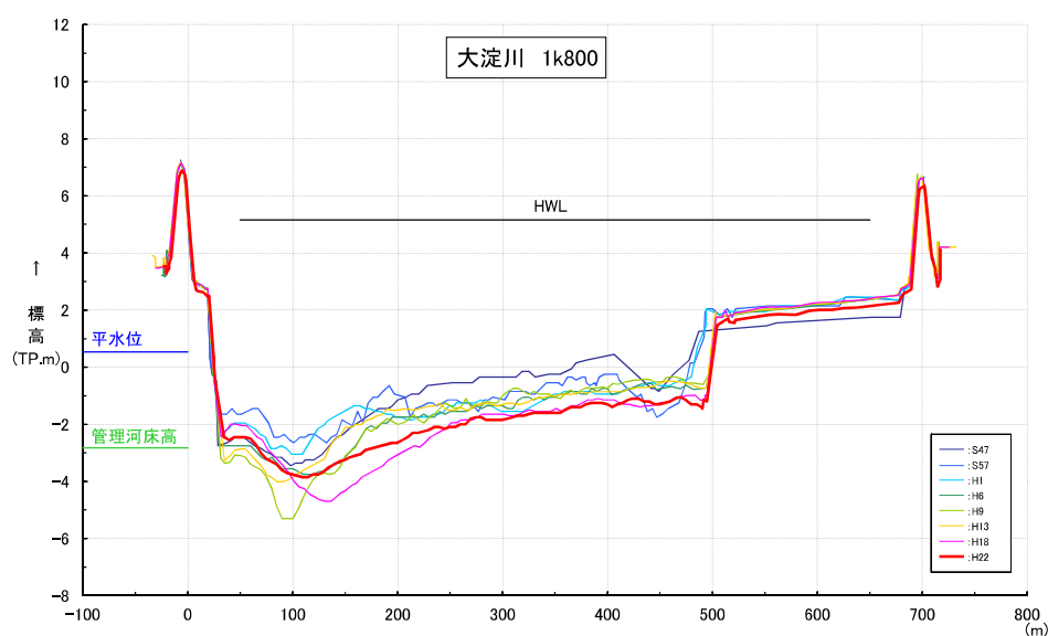
図 2-3(1) 代表横断面図（大淀川 1k800：河口付近）
