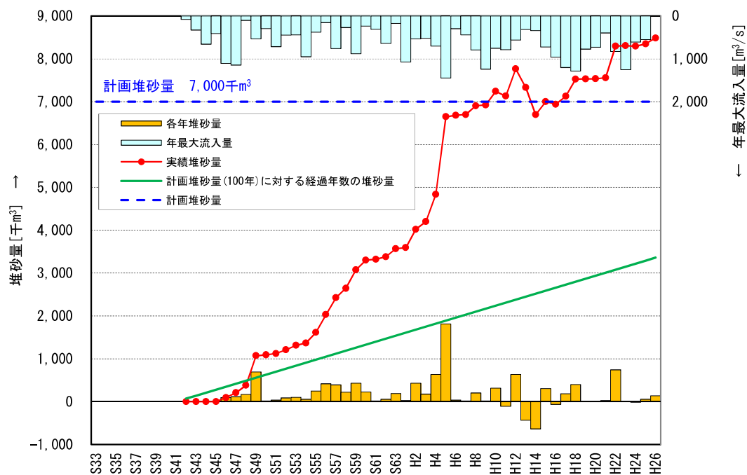
図 4-1 (1) 岩瀬ダムの堆砂状況
