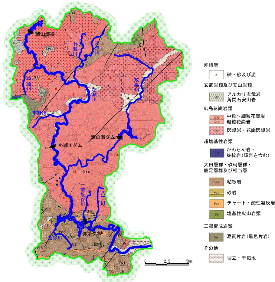
図-1.3.1 地質図
