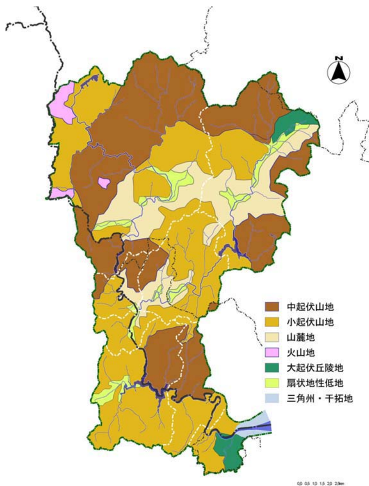
図-1.2.1 地形図
