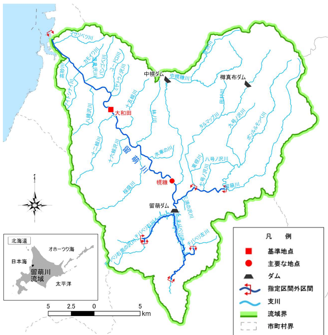
図 1-1 留萌川水系図
