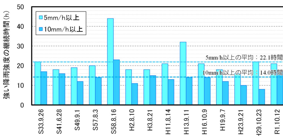
図 1-27 強い降雨強度の継続時間
