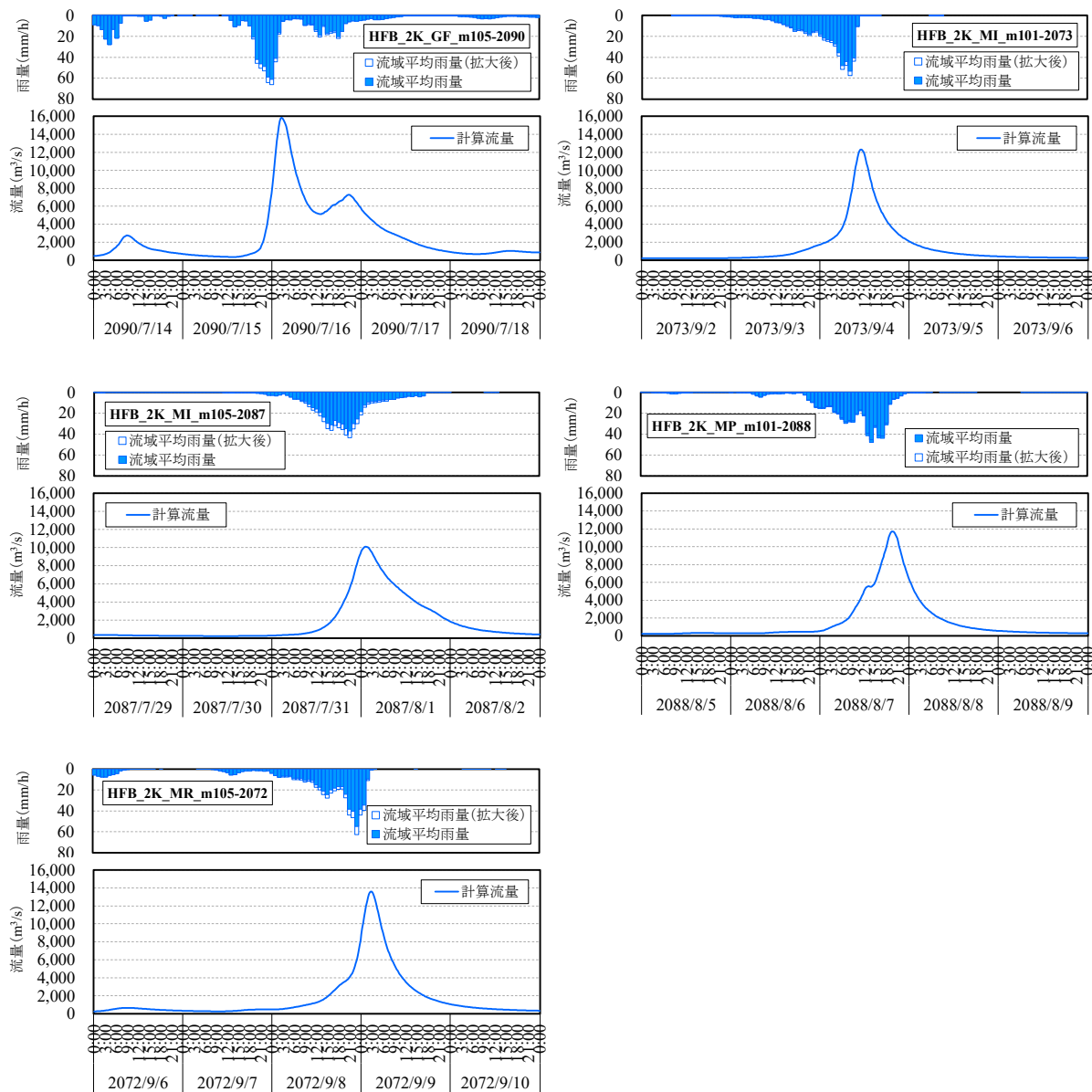
図 1-32 抽出した予測降雨波形のハイドログラフ(将来実験)
