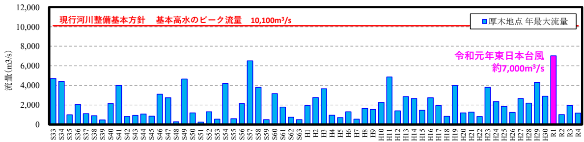
図 1-2 年最大流量(基準地点厚木)
