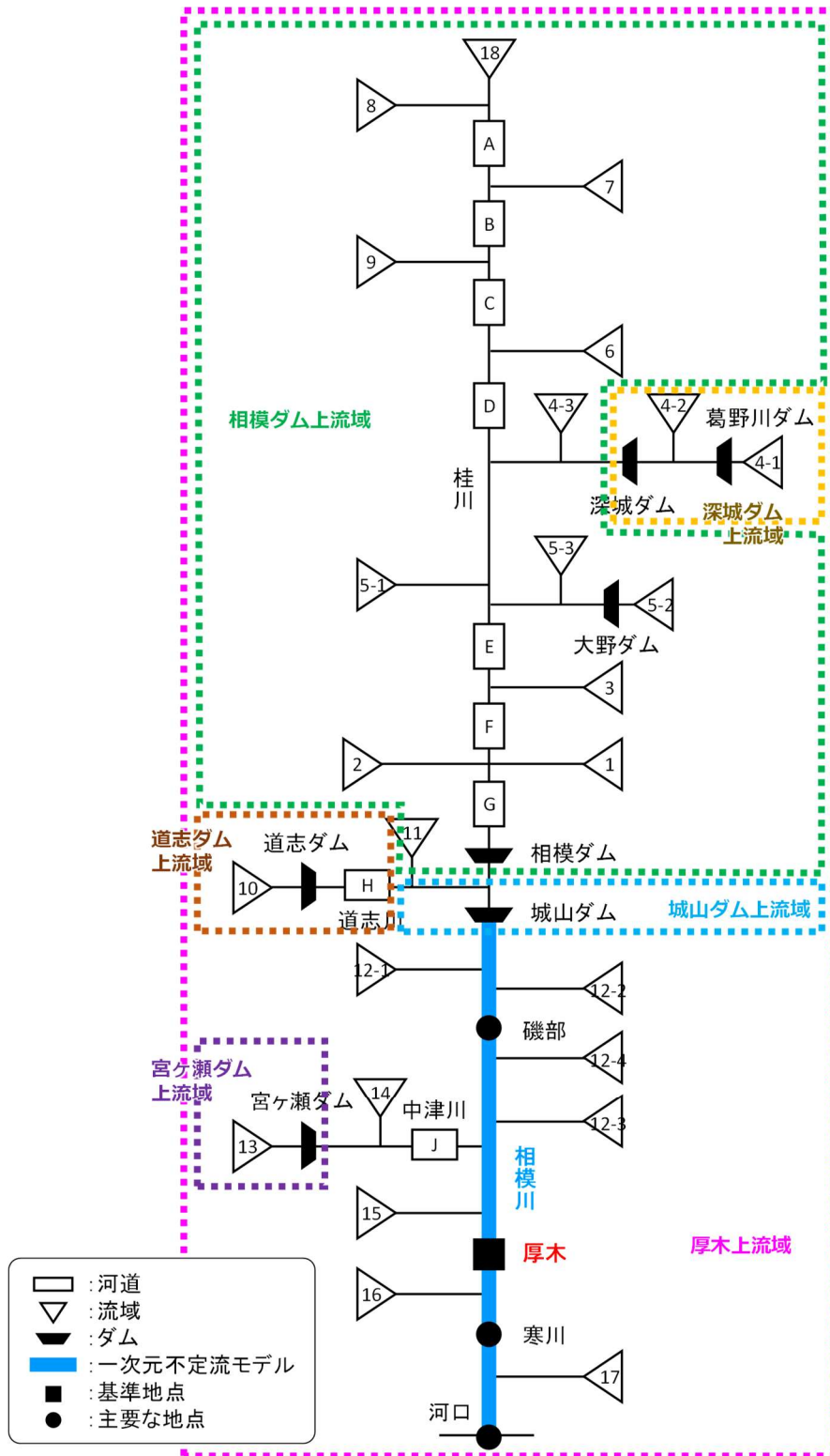
図 1-7 中流域分割図
