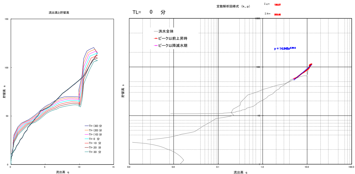
図 1-9 貯留高一流出高関係図
