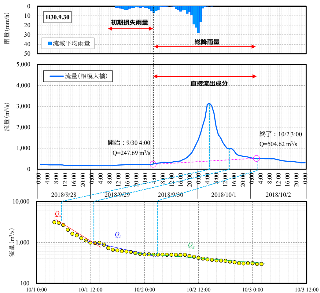
図 1-6 成分分離の事例(厚木地点、H30.9 洪水)
