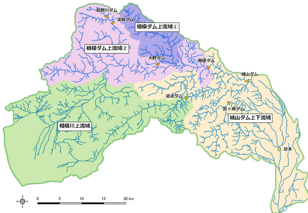
図 1-29 流域分割
