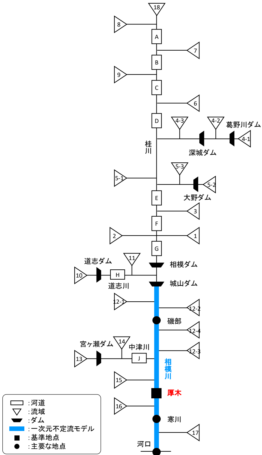
図 1-4 流出計算モデル模式図
