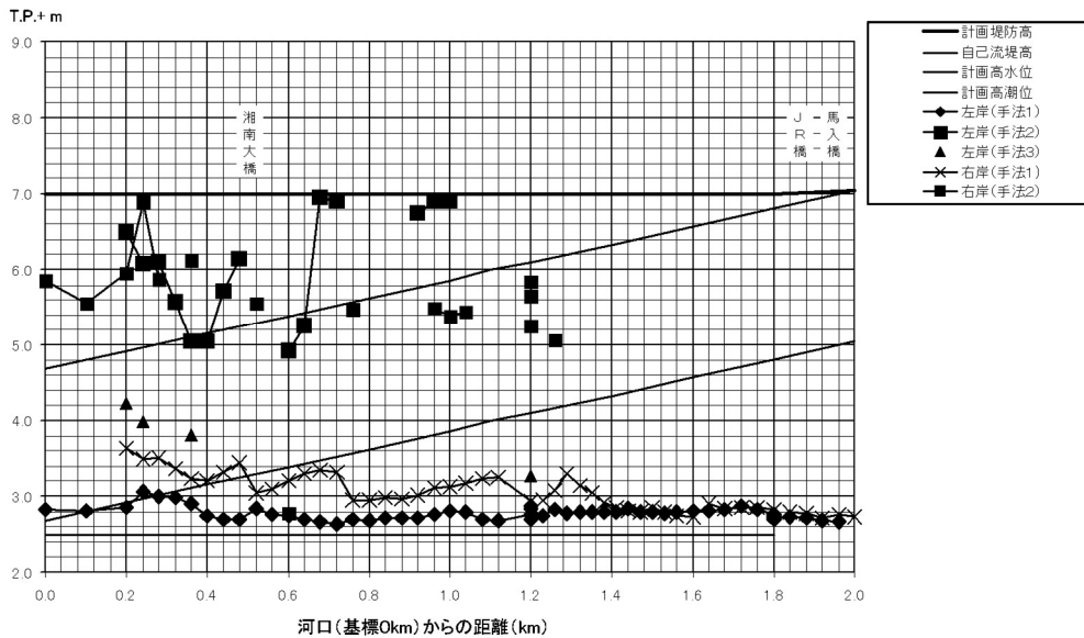
図 4-2 既往高潮計画における高潮堤防計画天端高
