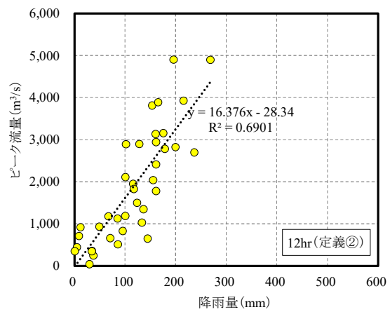
図 1-26 (1) ピーク流量と流域平均雨量の相関図【定義②】(1hr~12hr)
