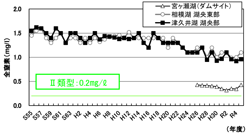
図 5-7 湖沼における水質の経年変化(全窒素)
