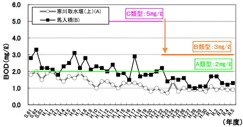
図 5-4 相模川下流部における水質の経年変化(BOD75%値)
