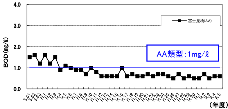
図 5-2 相模川上流部における水質の経年変化 (BOD75%値)
