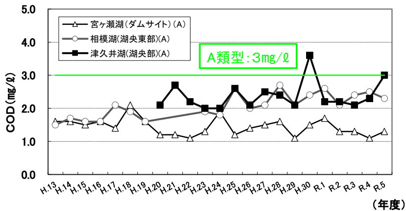
図 5-6 湖沼における水質の経年変化(COD75%値)
