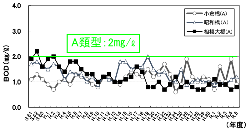
図 5-3 相模川中流部における水質の経年変化 (BOD75%値)
