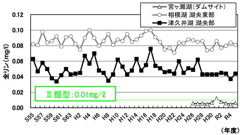
図 5-8 湖沼における水質の経年変化(全リン)
