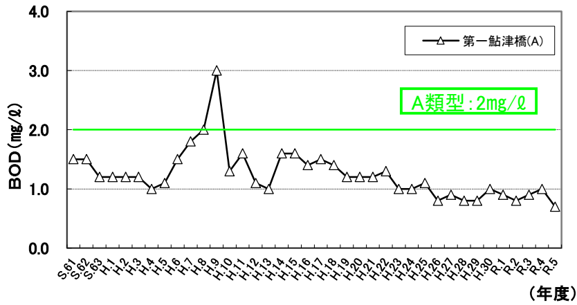
図 5-5 相模川支川(中津川)における水質の経年変化(BOD75%値)
