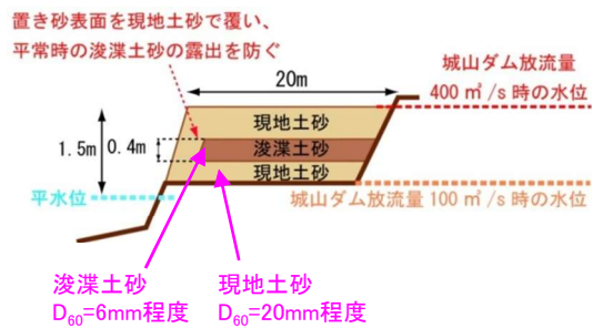
置き砂の設置方法
