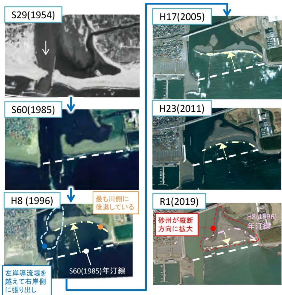
図 5-1 河口砂州の位置の変化
