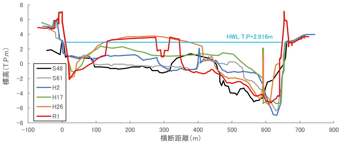
図 5-3 相模川 0.2k 経年変化横断面図
