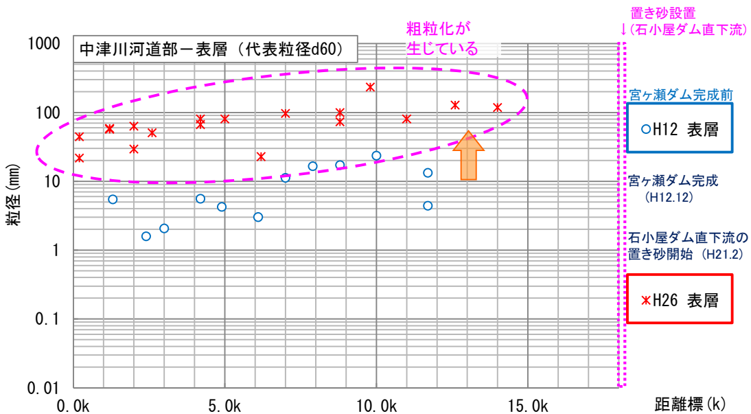
図 4-8 代表粒径縦断面図(中津川)
