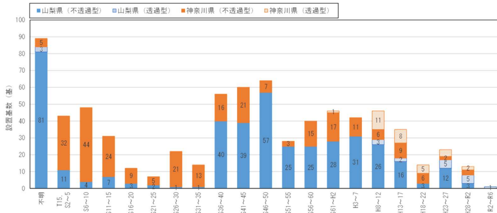
図 2-2 砂防堰堤の設置基数の推移(大正15年～令和6年)
