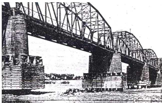
図 4-102 砂利採取によって橋脚が浮き上がった旧相模橋
