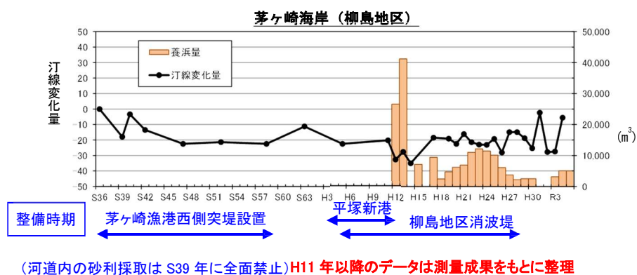
図 6-11 養浜量と汀線変化量
