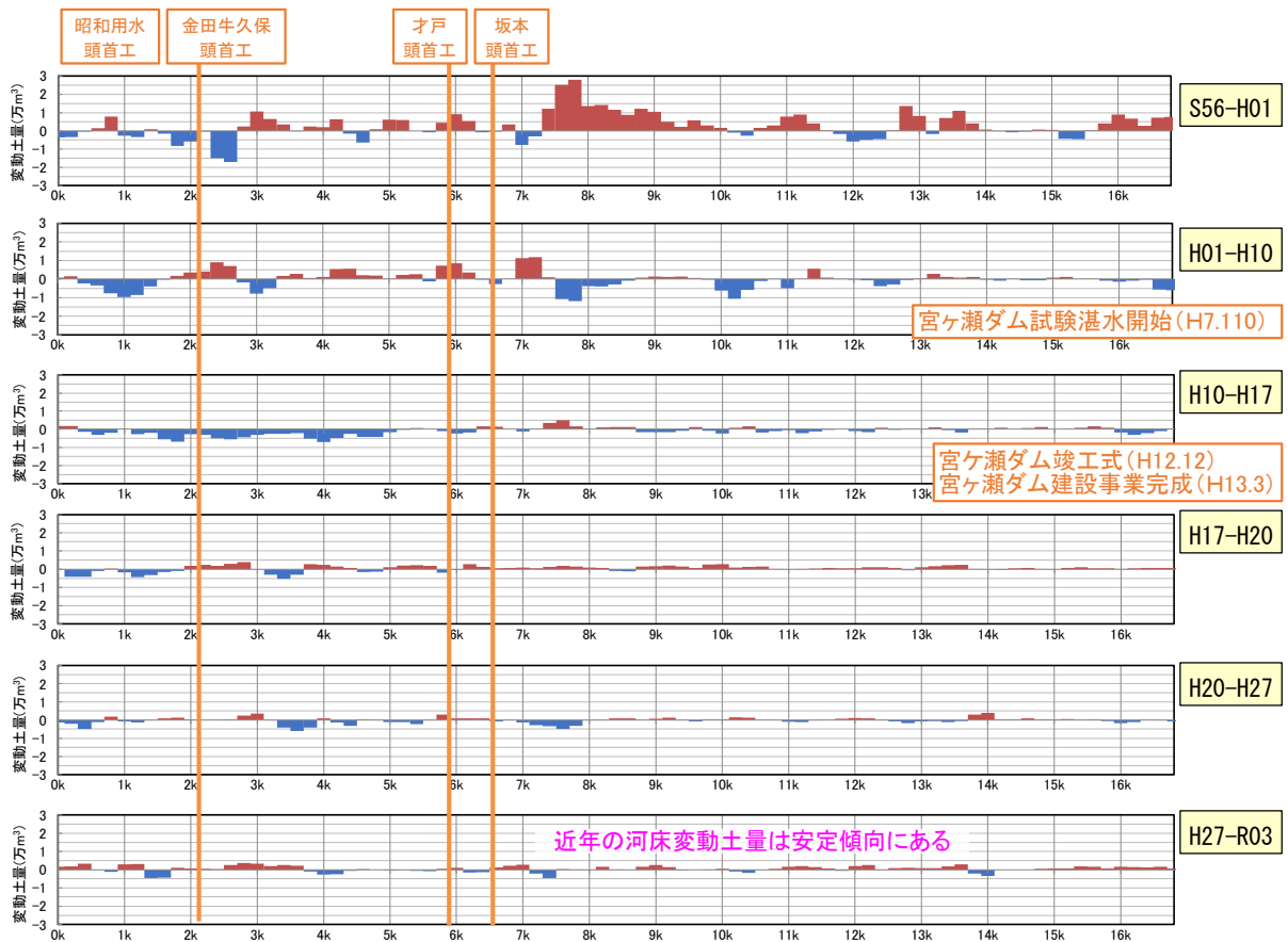
図 4-2 中津川 河床変動土量縦断面図
