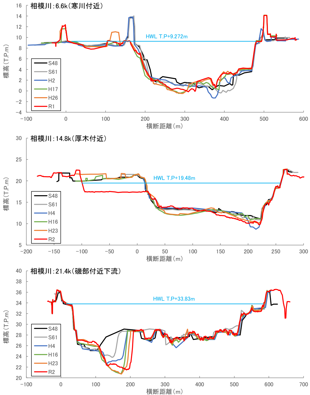
図 4-5 経年変化横断図(相模川)
