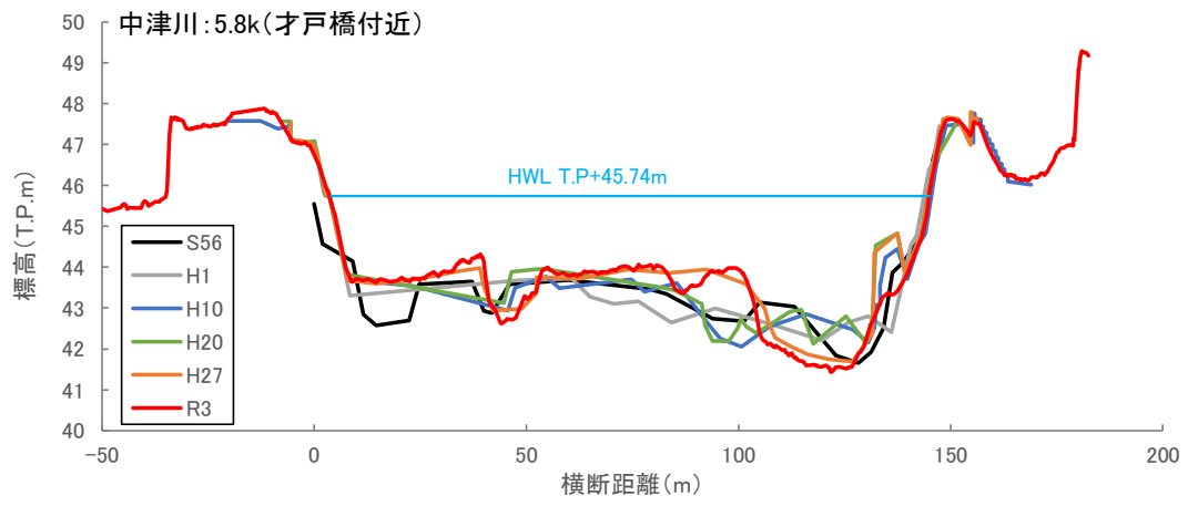
図 4-6 経年変化横断面図(中津川)
