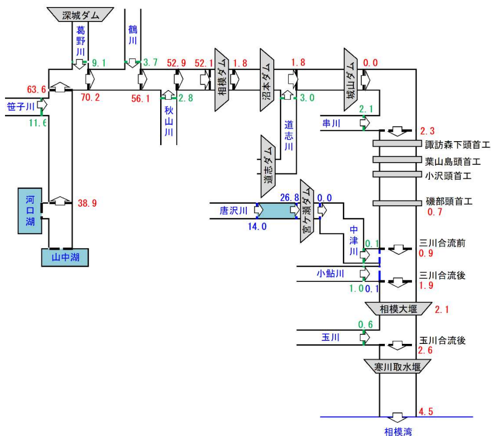
図 4-9 年平均通過土砂量
