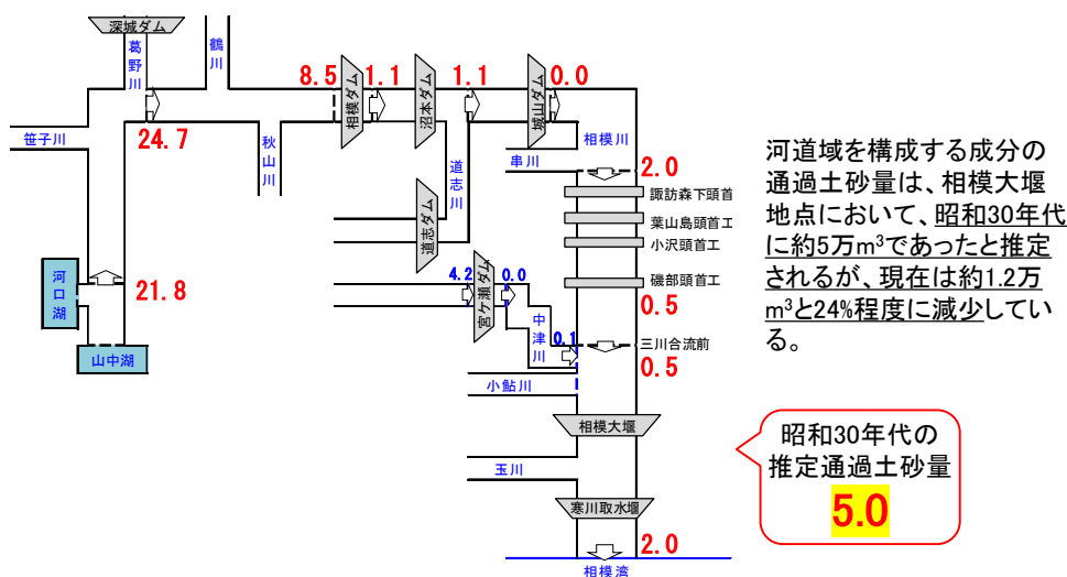
図 4-10 河道域構成成分 ( d_{60}=1\sim70\text{mm} ) の土砂動態
