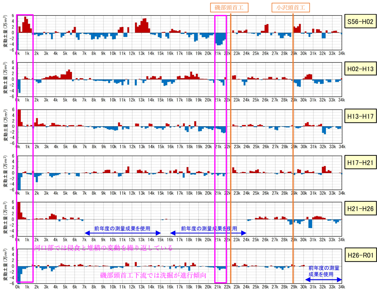
図 4-1 相模川 河床変動土量縦断図
