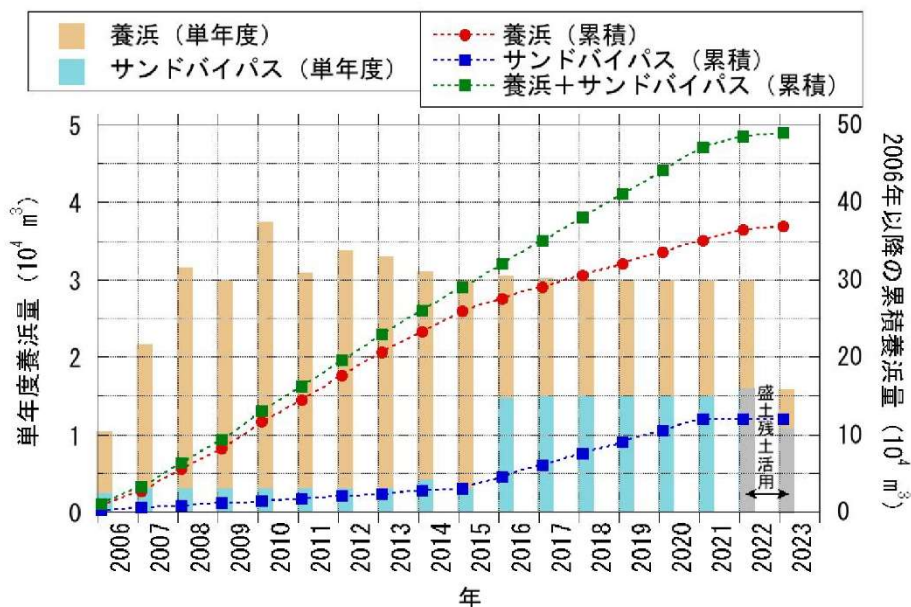
図 6-10 養浜及びサンドバイパスの量(神奈川県提供)
