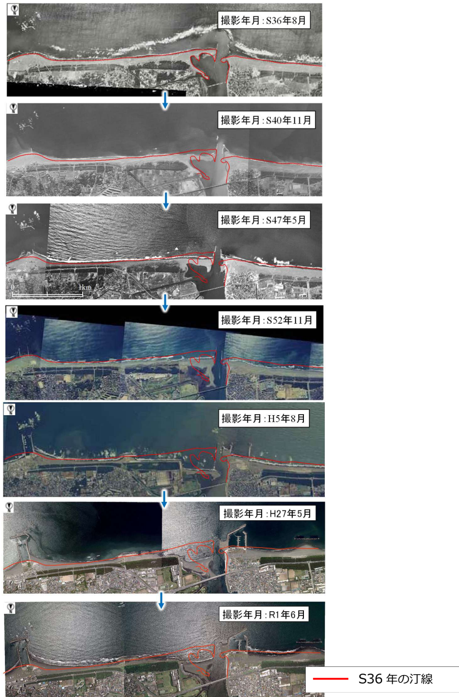
図 5-4 汀線位置の変遷
