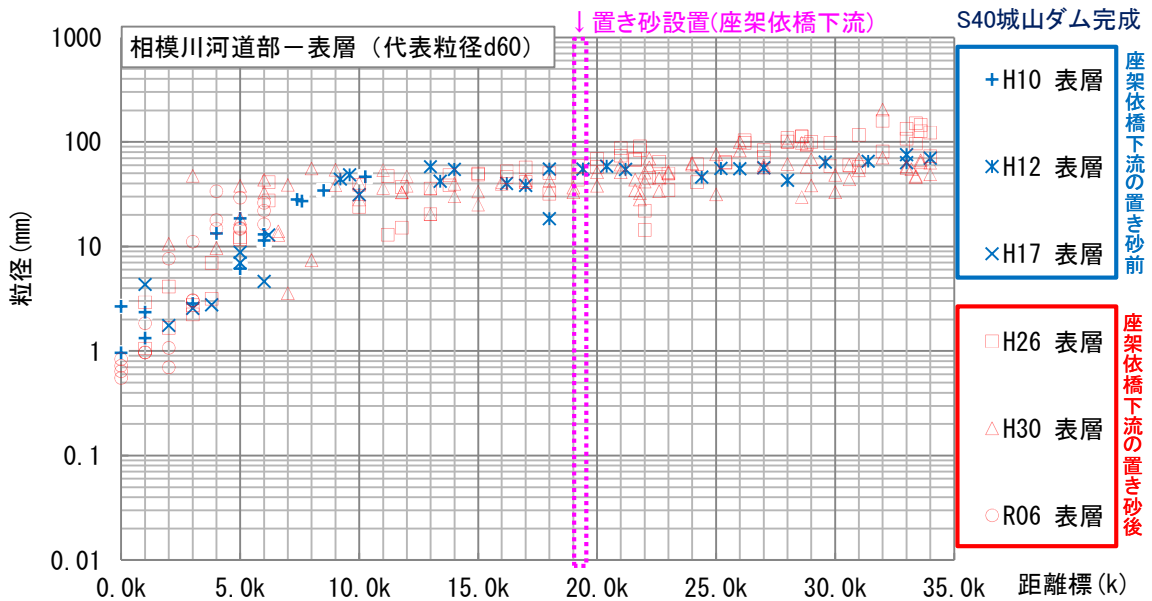
図 4-7 代表粒径縦断面図(相模川)
