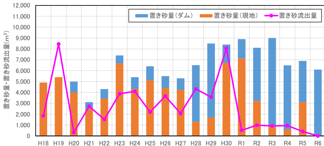
図 6-4 相模川置き砂試験施工の置き砂量(平成 18 年~令和 6 年)
