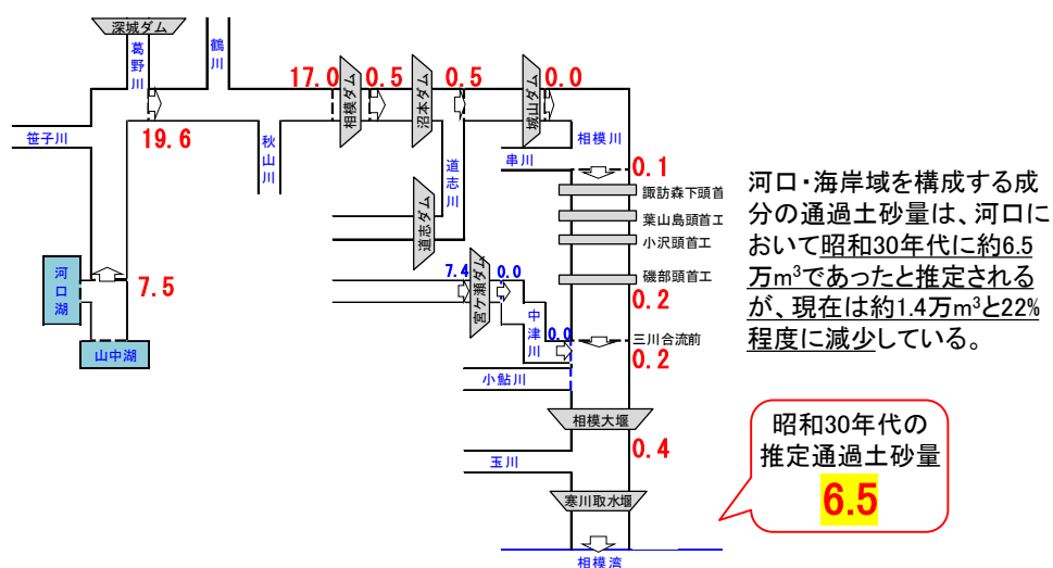
図 4-11 河道域構成成分 ( d_{60}=0.2\sim1\text{mm} ) の土砂動態
