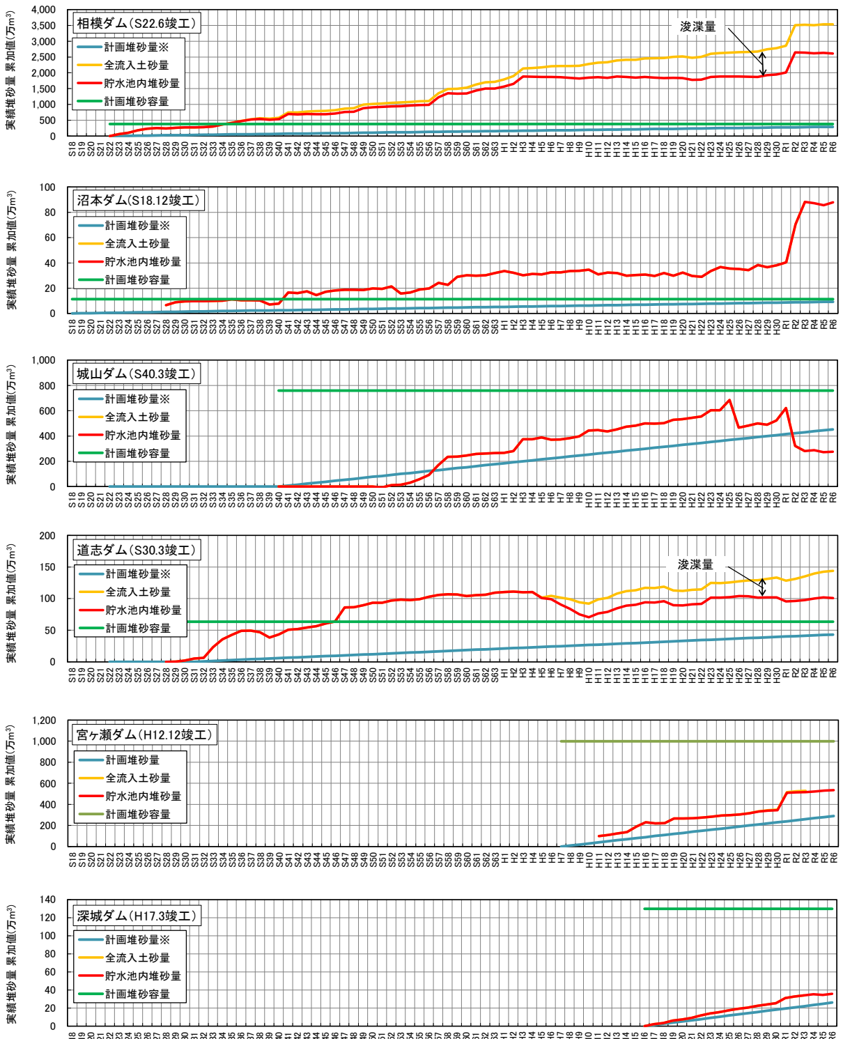
図 3-4 ダムの堆砂状況(各ダムの竣工以降～令和4年度)
