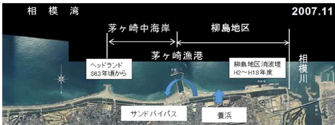
図 5-5 海岸域の侵食対策(構造物対策及び養浜)
