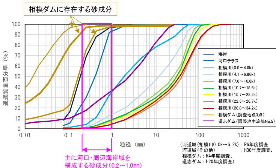
図 3-3 相模ダム浚渫土と河道域、河口・周辺海岸域の河床構成材料
