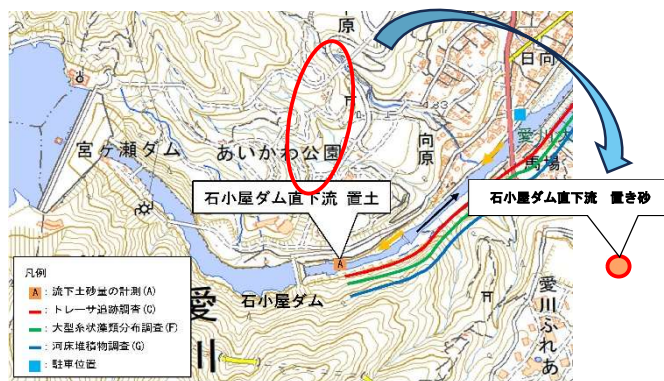
図 6-7 中津川置き砂実施箇所(中津川 18.8k 左岸)
