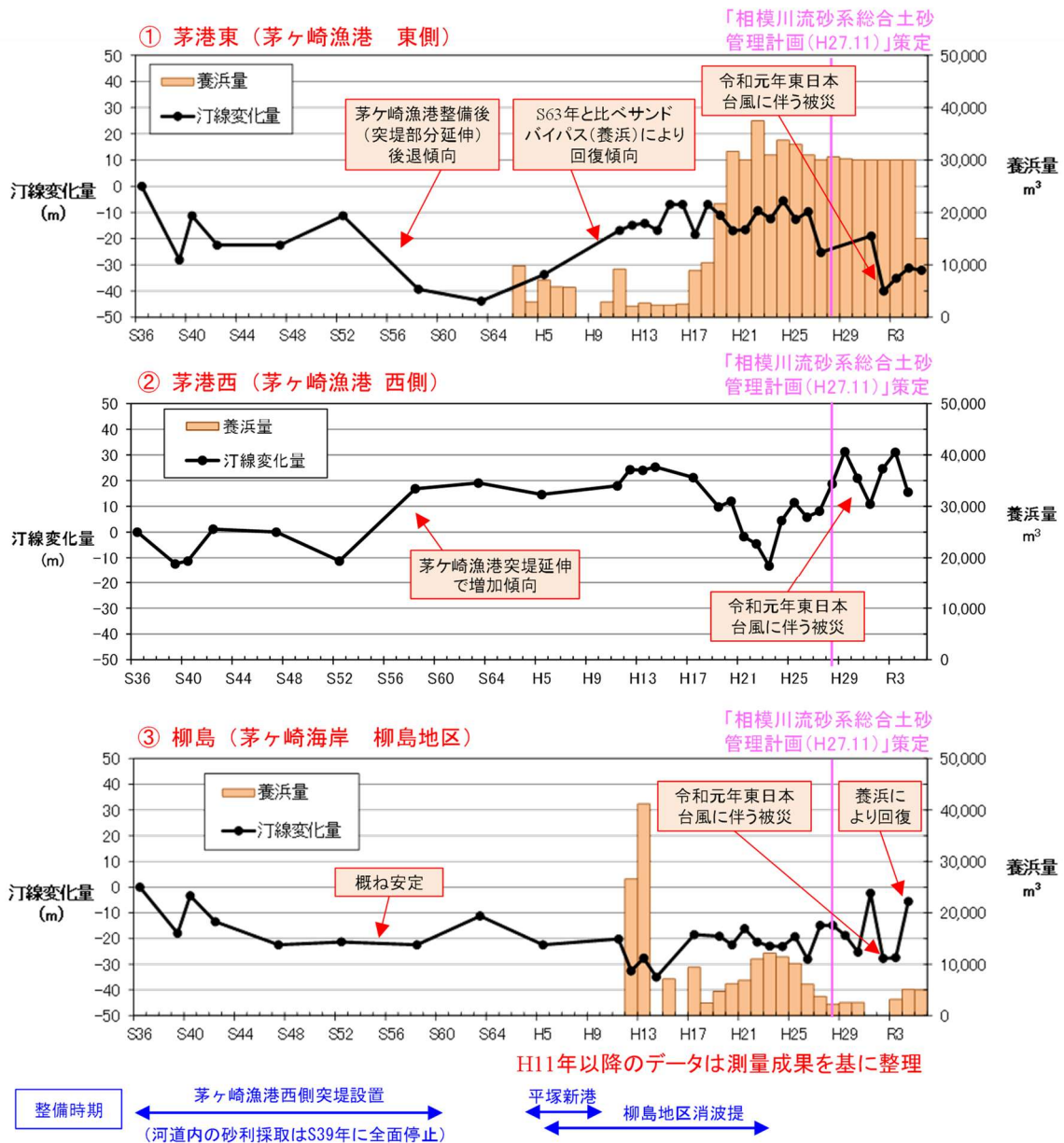
図 5-7 航空写真に基づき算出した汀線変化量(相模川河口～茅ヶ崎漁港)
