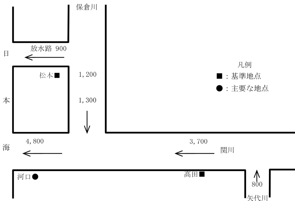
関川計画高水流量図（単位： \text{m}^3/\text{s} ）
