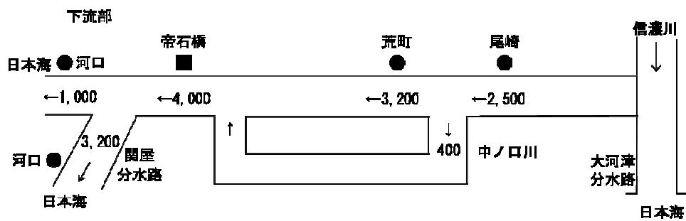
下流部計画高水流量図 (単位：m 3 /s)
