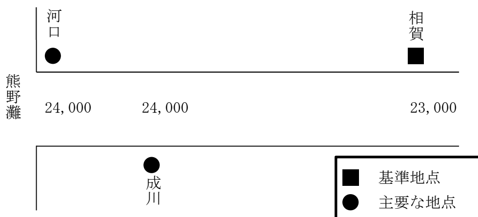
熊野川計画高水流量図 (単位 : \text{m}^3/\text{s} )
