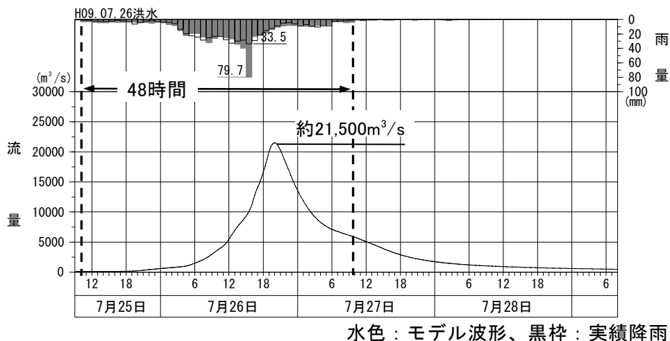
図 4-9 モデル降雨による流出解析結果（平成 9 年 7 月洪水確率 48 時間雨量）
