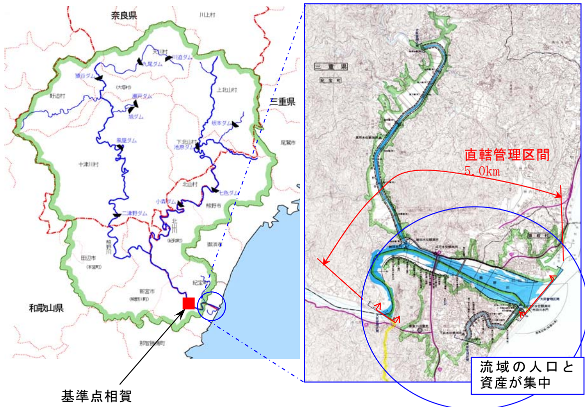
図 4-3 直轄管理区間と基準点相賀位置図
