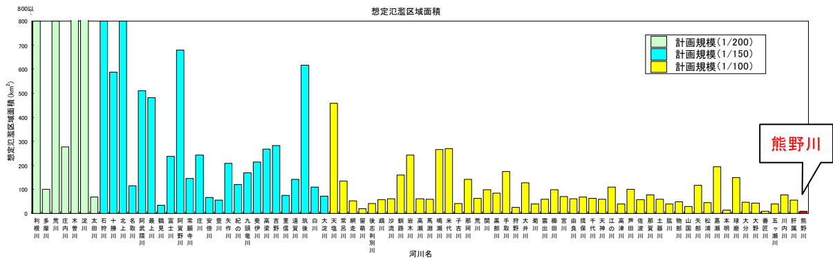
図 4-5(1) 熊野川流域の想定氾濫区面積
