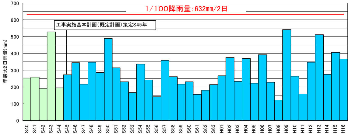
図 4-1 年最大 2 日雨量 (相賀地点上流域平均)
