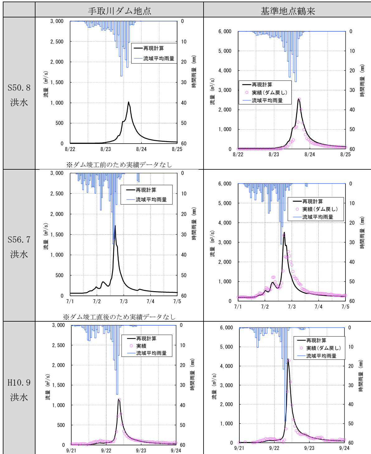
図 1-12(1) 再現計算結果
