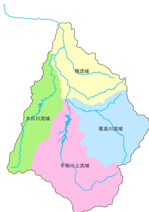
図 1-20 検討対象地域位置図
