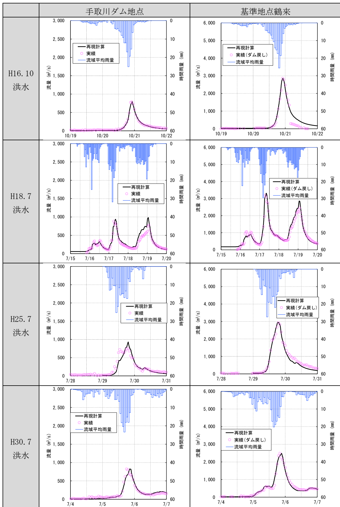
図 1-12(2) 再現計算結果
