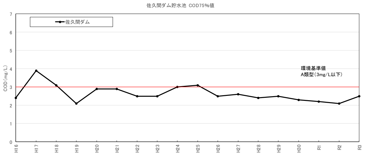
図 5.5 天竜川水系湖沼の水質変化(COD)
