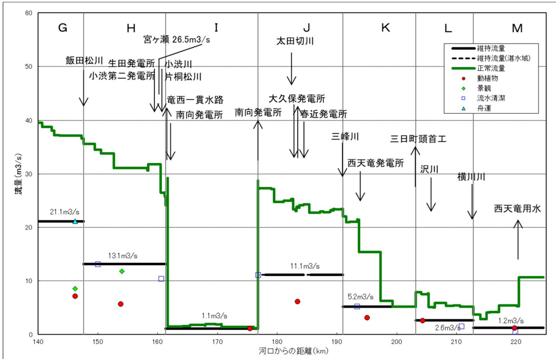
図 6.3 天竜川正常流量縦断図(上流)(3/4)
