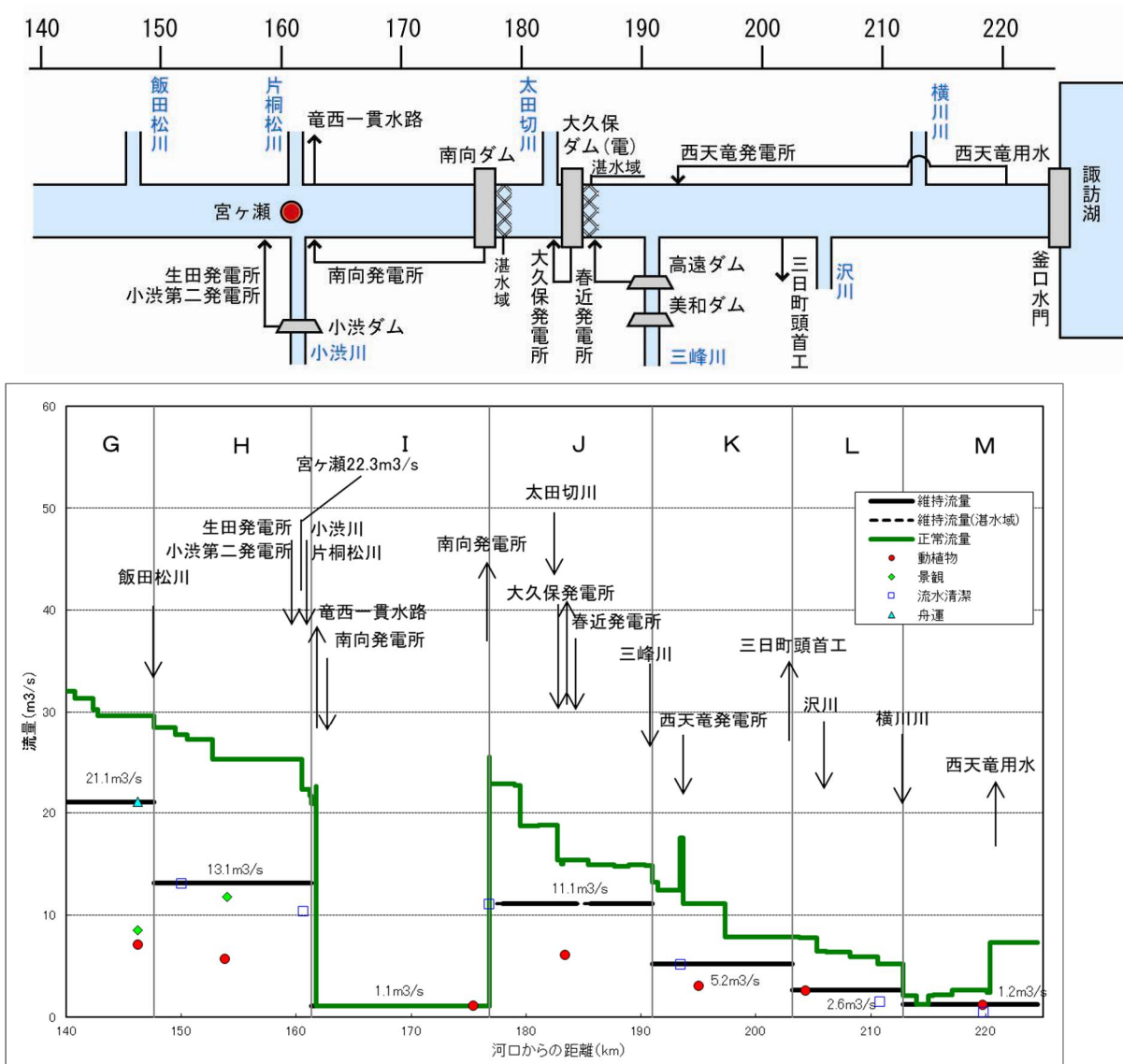
図 6.4 天竜川正常流量縦断図(上流)(4/4)
