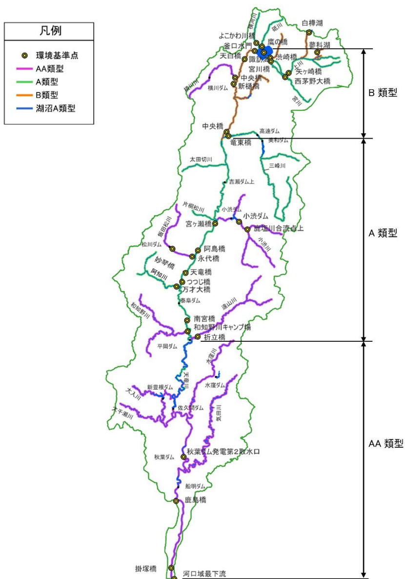
図 5.1 類型指定の範囲
