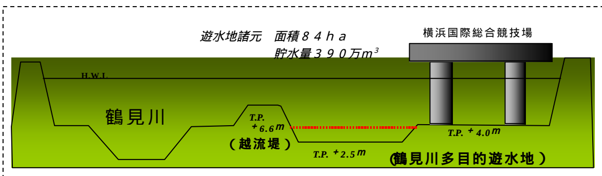
図 4-3-10 鶴見川多目的遊水地の諸元等 出典: 京浜河川事務所
