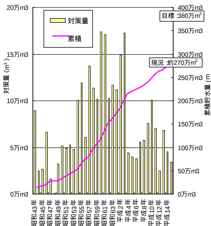
図 4-3-12 鶴見川流域の防災調整池の推移
