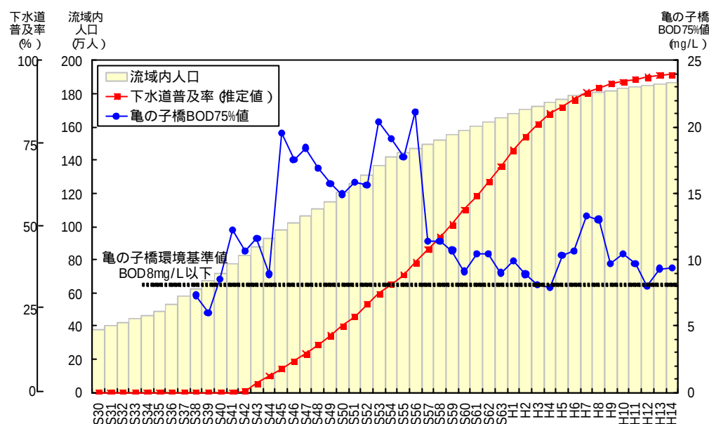
図 6-3-8. 流域内の人口、下水道普及率と水質の変遷
