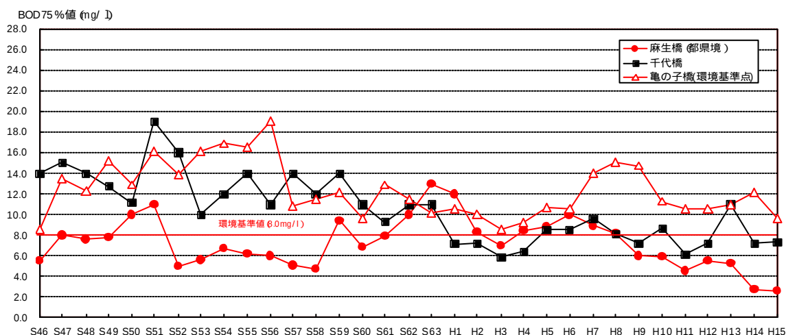
図 6-3-3 鶴見川本川の環境基準 D 類型指定区間における BOD 経年変化
