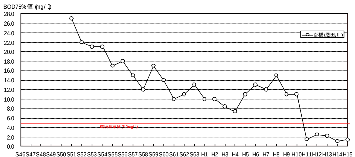
図 6-3-5 支川 (恩田川) の環境基準 C 類型指定区間における BOD の経年変化 出典：京浜河川事務所
