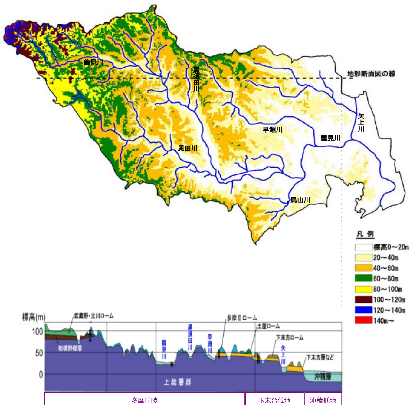
図 1-2-1 地形図と地形断面図
