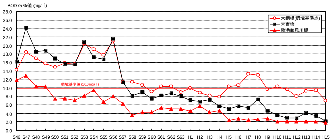
図 6-3-2 鶴見川本川の環境基準 E 類型区間における BOD の経年変化
