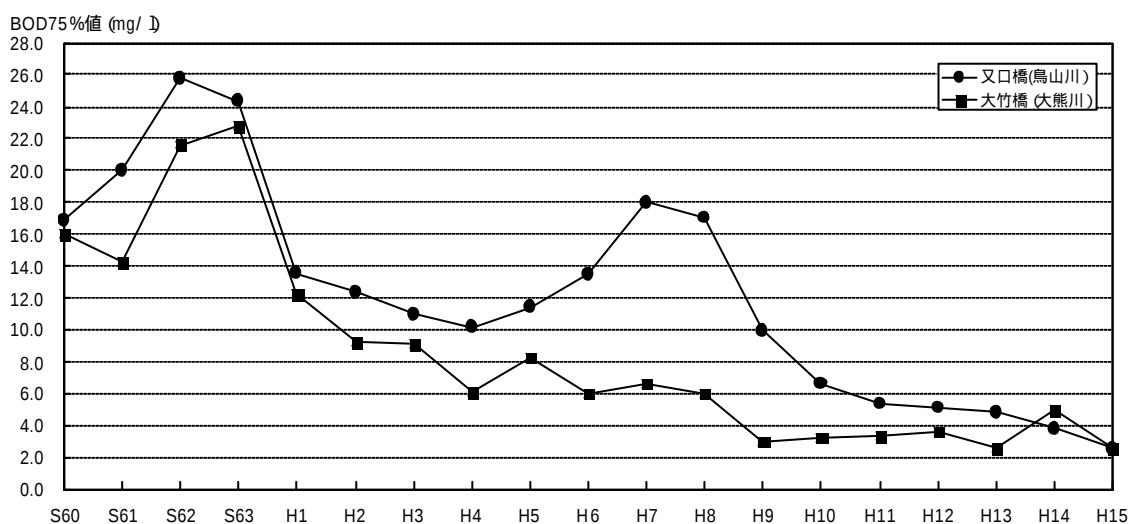
図 6-3-7 支川(鳥山川・大熊川)における BOD の経年変化 出典：京浜河川事務所
