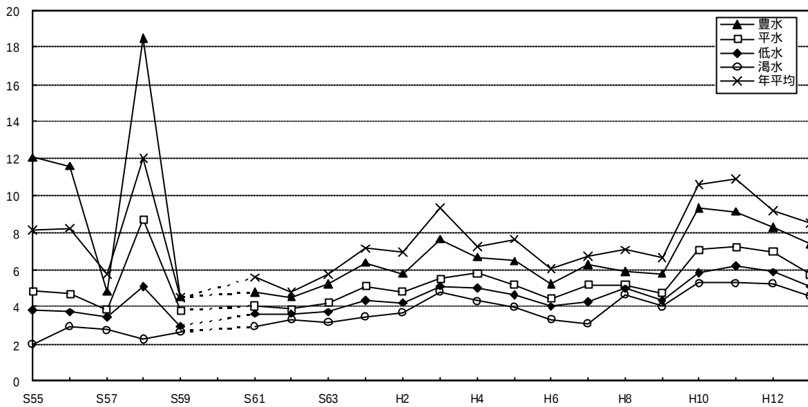
図 6-1-1 鶴見川落合橋の流況の経年変化
