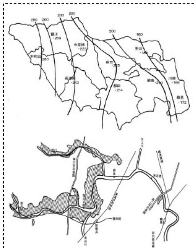
図 4-2-3 昭和 51 年 6 月洪水 - 総雨量等雨量線図と洪水浸水区域図 - 出典: 鶴見川流域誌 / 河川編、京浜河川事務所
