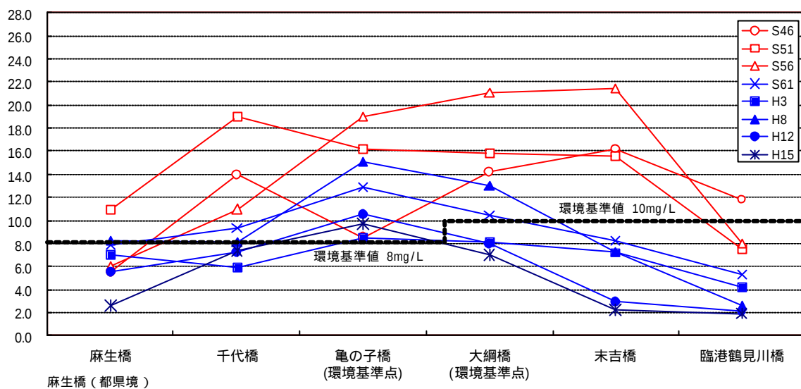
図 6-3-4 鶴見川本川の BOD75% 値の縦断変化 出典：京浜河川事務所
