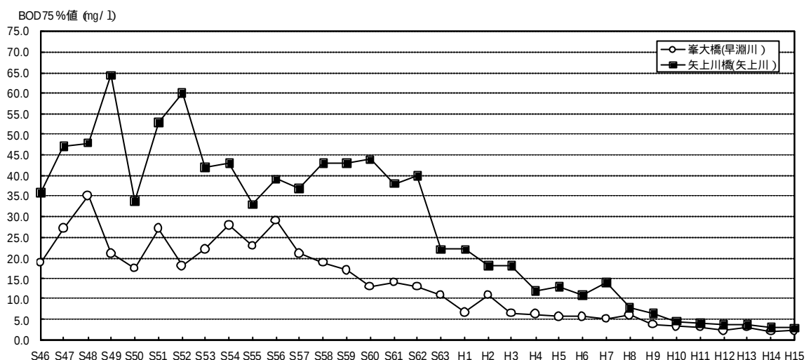
図 6-3-6 支川(早淵川・矢上川)における BOD の経年変化 出典：京浜河川事務所
