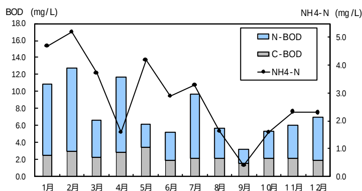
図 6-3-9 亀の子橋におけるBODの内訳 (平成 15 年)
