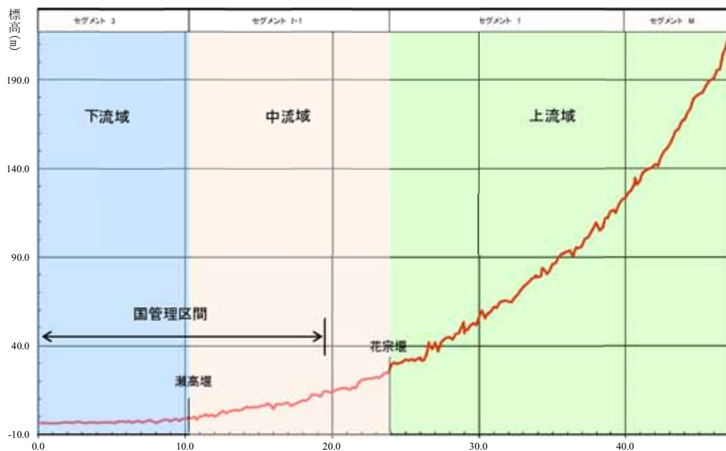
図-8.1 矢部川の河床勾配（最深河床高）
