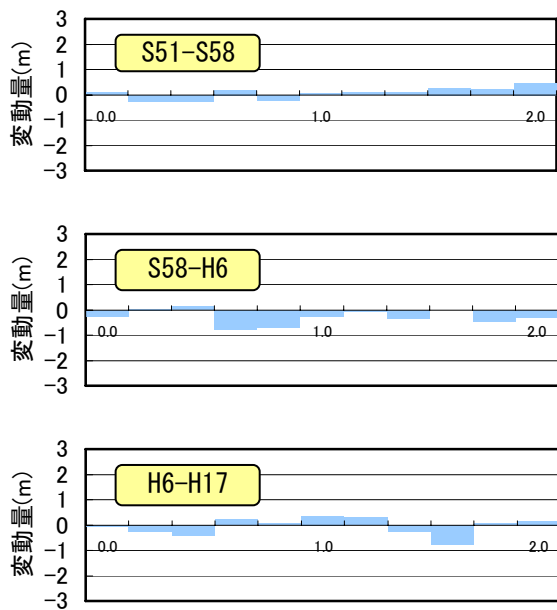
図 8.6 曽我川平均河床変動量の縦断変化図 昭和 51 年～平成 17 年
