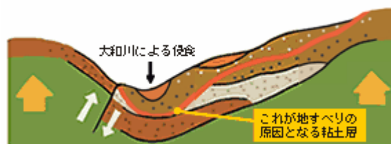
図 4.17 亀の瀬地質
