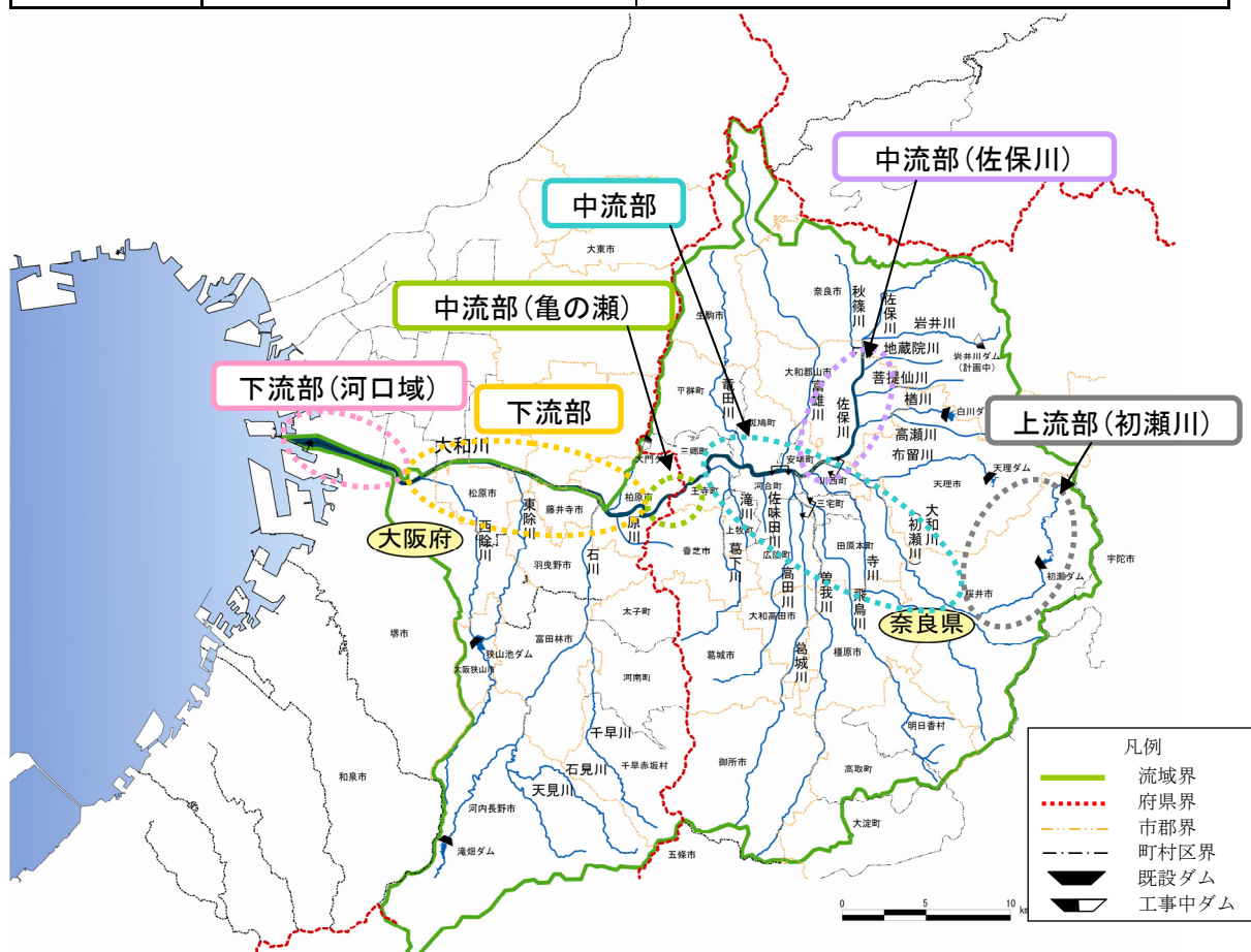
図 2.2 大和川の自然環境区分
