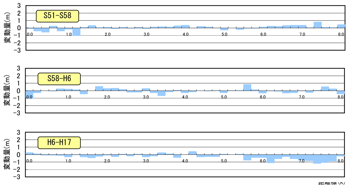
図 8.5 佐保川平均河床変動量の縦断変化図 昭和 51 年～平成 17 年
