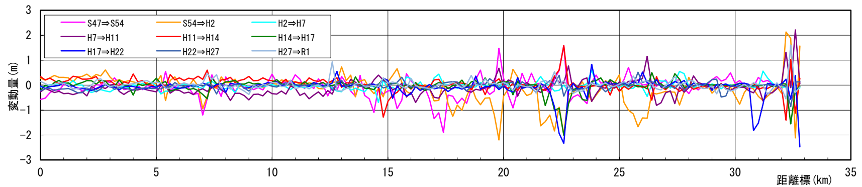
図 4-2 平均河床変動量縦断面図(吉井川)
