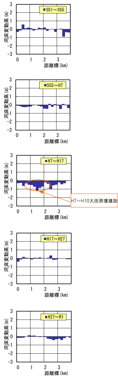
図 4-6 低水路内河床変動高経年変化図(金剛川)
