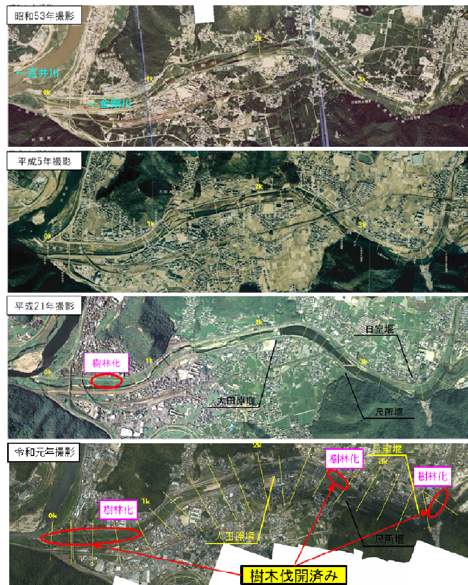
図 4-11 (4) 河道の変遷 (航空写真)
