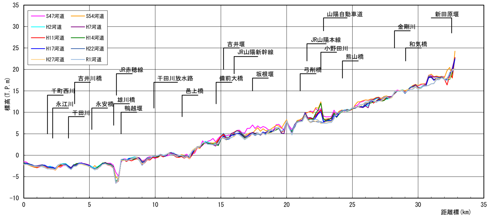
図 4-1 低水路平均河床高縦断面図(吉井川)
