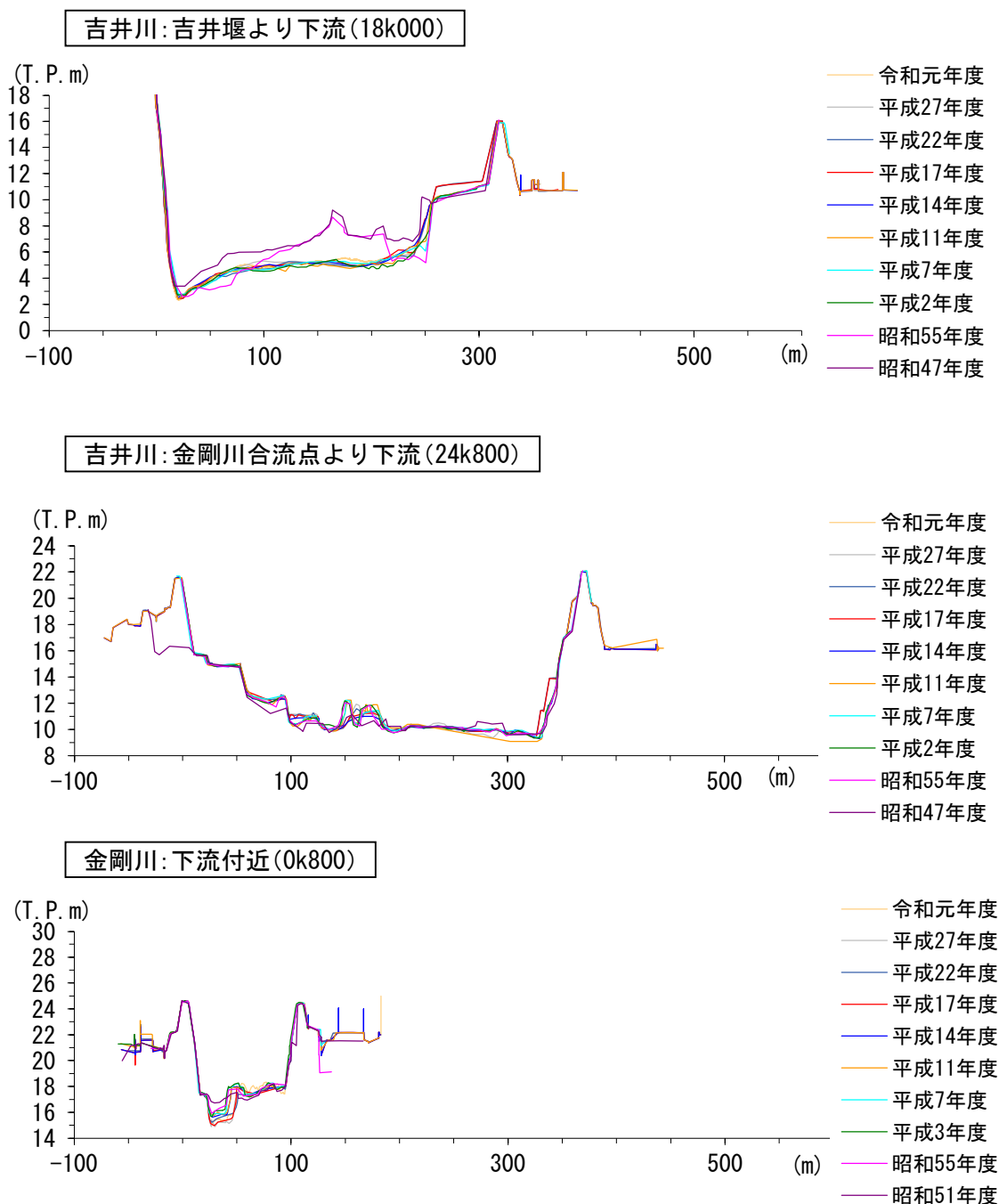
図 4-7 経年変化横断図
