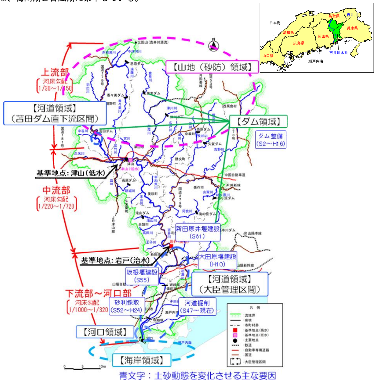
図 1-1 吉井川水系流域図
