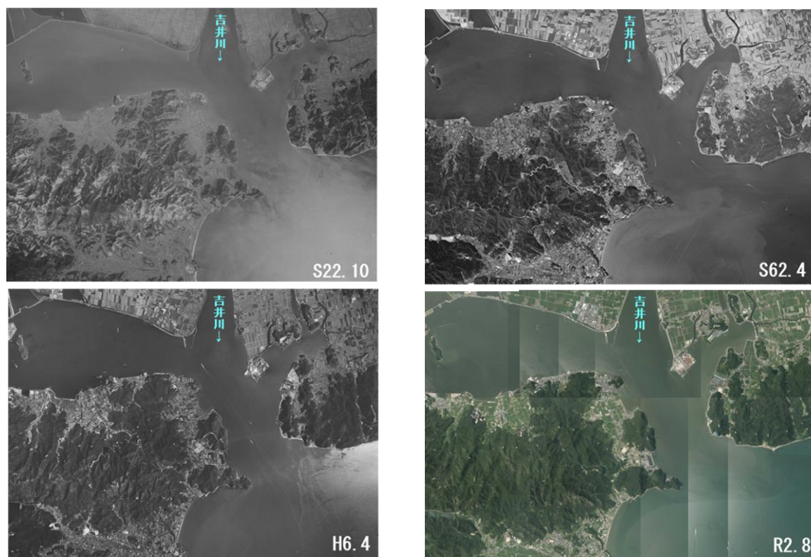
図 6-1 汀線の変遷
