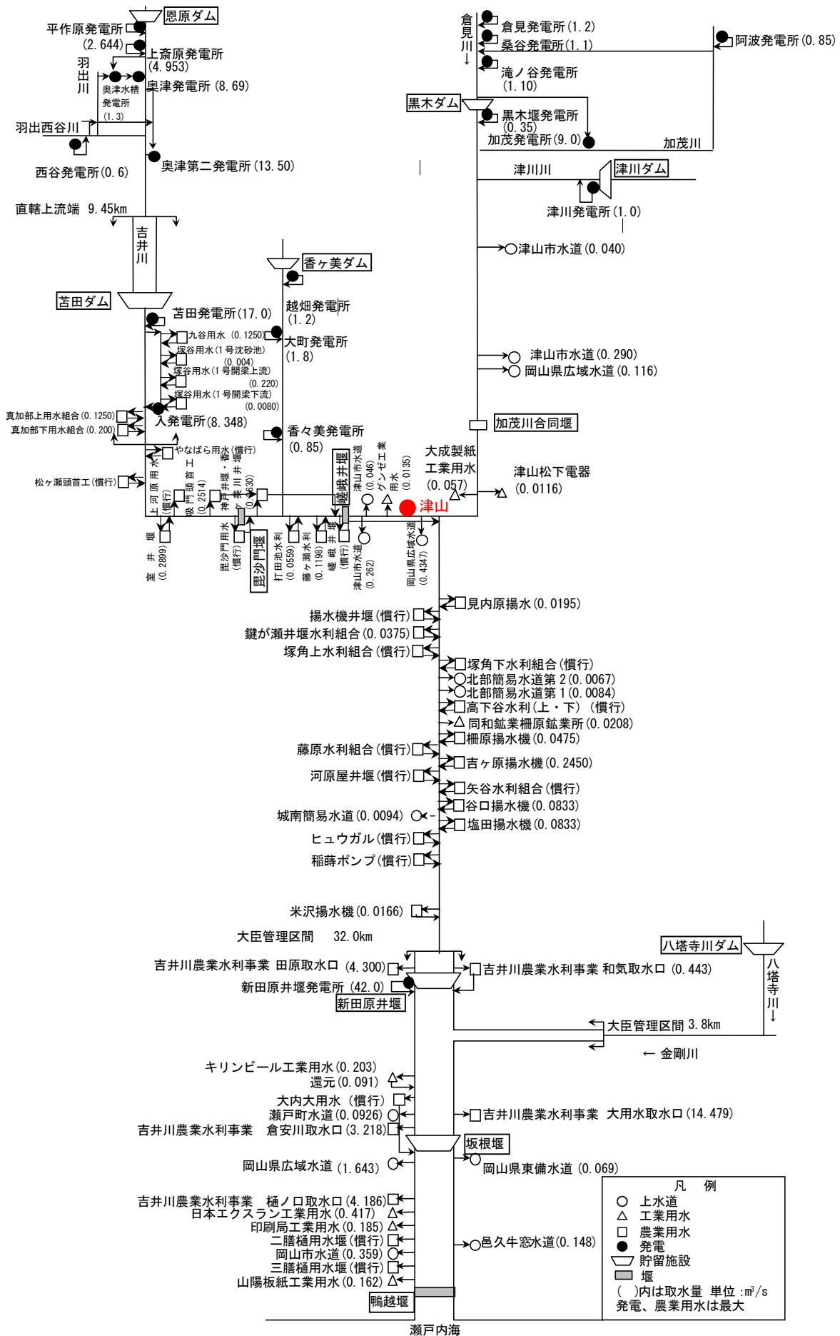
図-5.1.5 水利模式図
