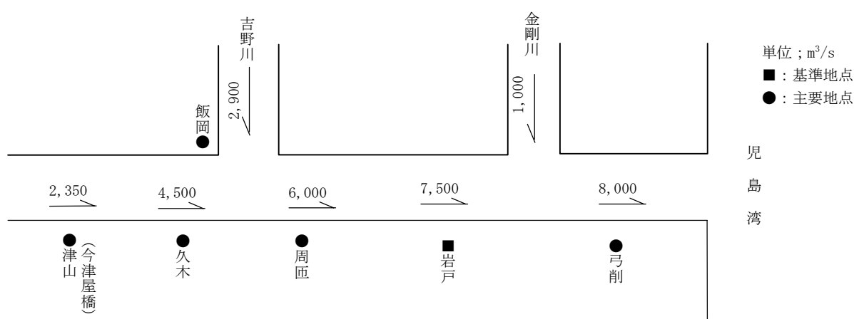
図-4.2.2 流量配分図 (吉井川水系工事实施基本計画 : 昭和 48 年)
