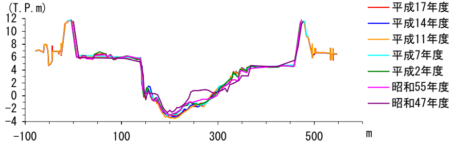
図-8.2.2(1) 河床横断面経年変化図(吉井川：12K400)
