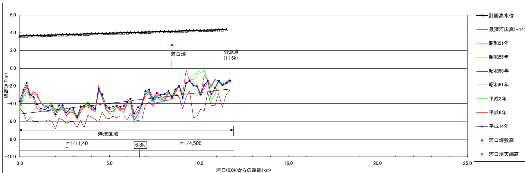
図-8.7(2) 今切川 平均河床高
