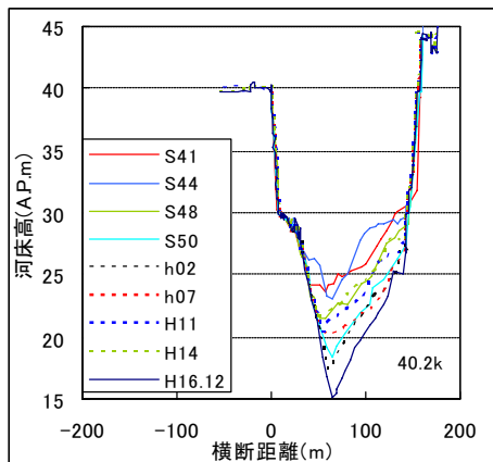
図－8. 2 (2) 横断形状の経年変化 (40. 2k)
