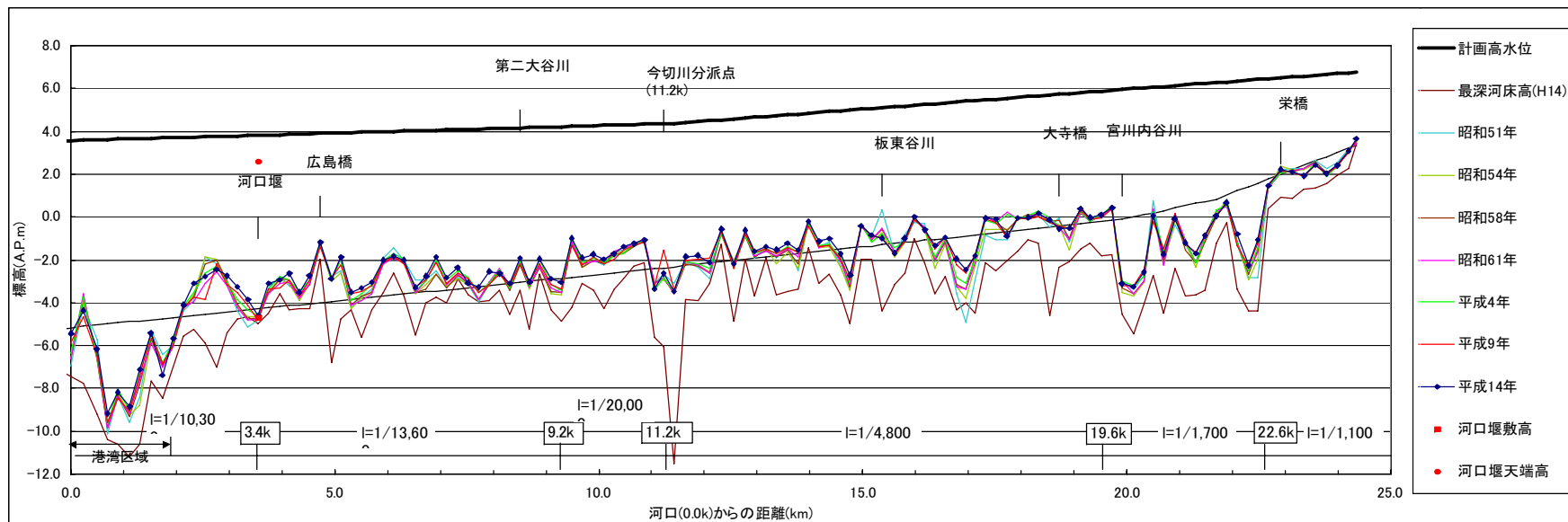
図-8.7(1) 旧吉野川 平均河床高
