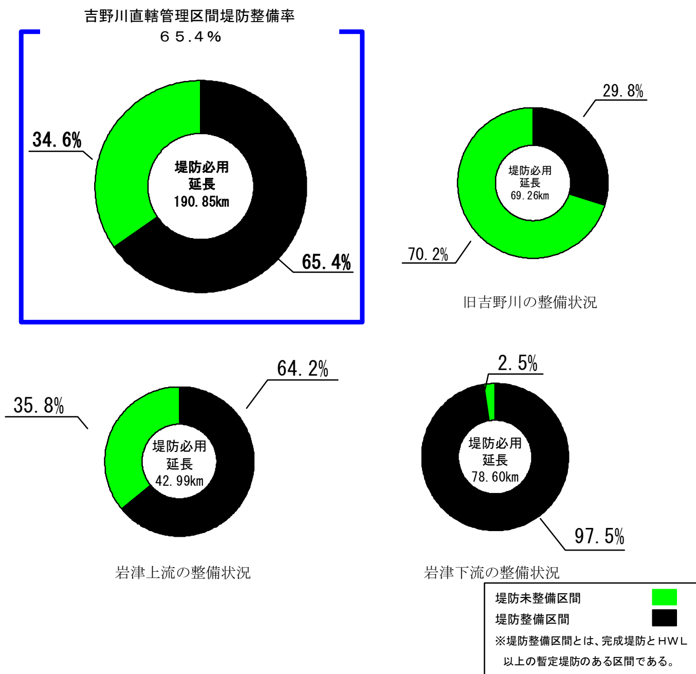
図-4.17(2) 吉野川直轄管理区間の堤防整備状況(平成17年3月現在)(2)
