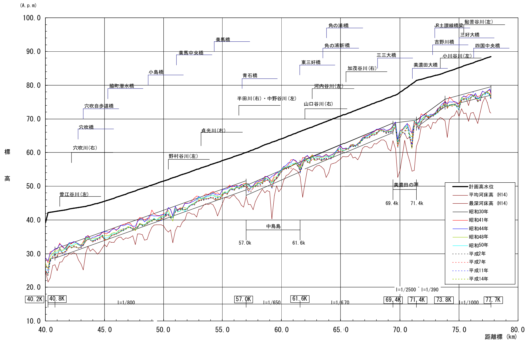
図-8.3(2) 吉野川上流 平均河床高
