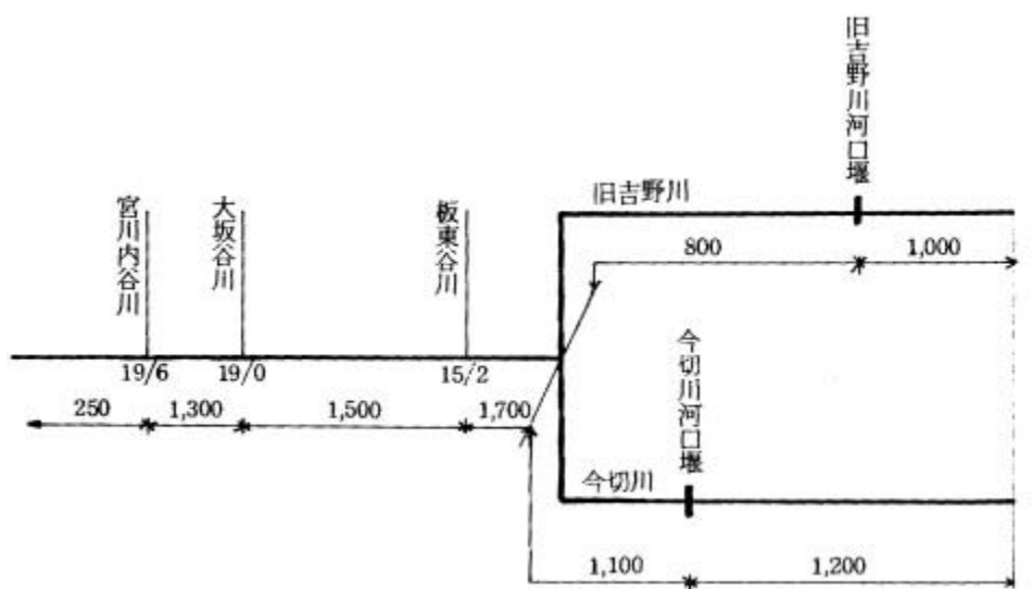
図-4. 16(3) S57工実(1/100規模)
