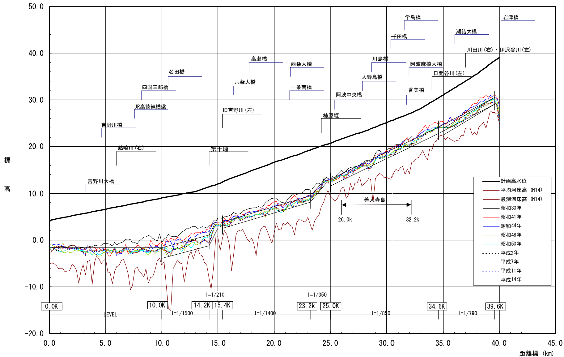
図-8.3(1) 吉野川下流 平均河床高
