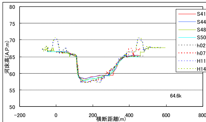
図－8. 2 (3) 横断形状の経年変化 (64. 6k)
