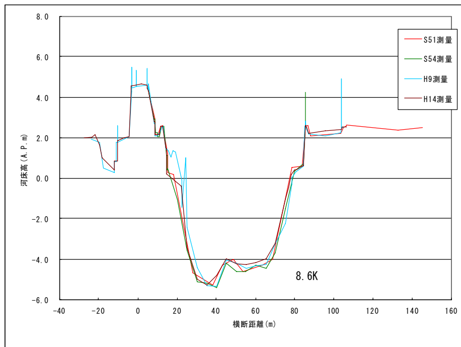
図8. 6(1) 横断形状の経年変化（馬詰橋付近8. 6k）
