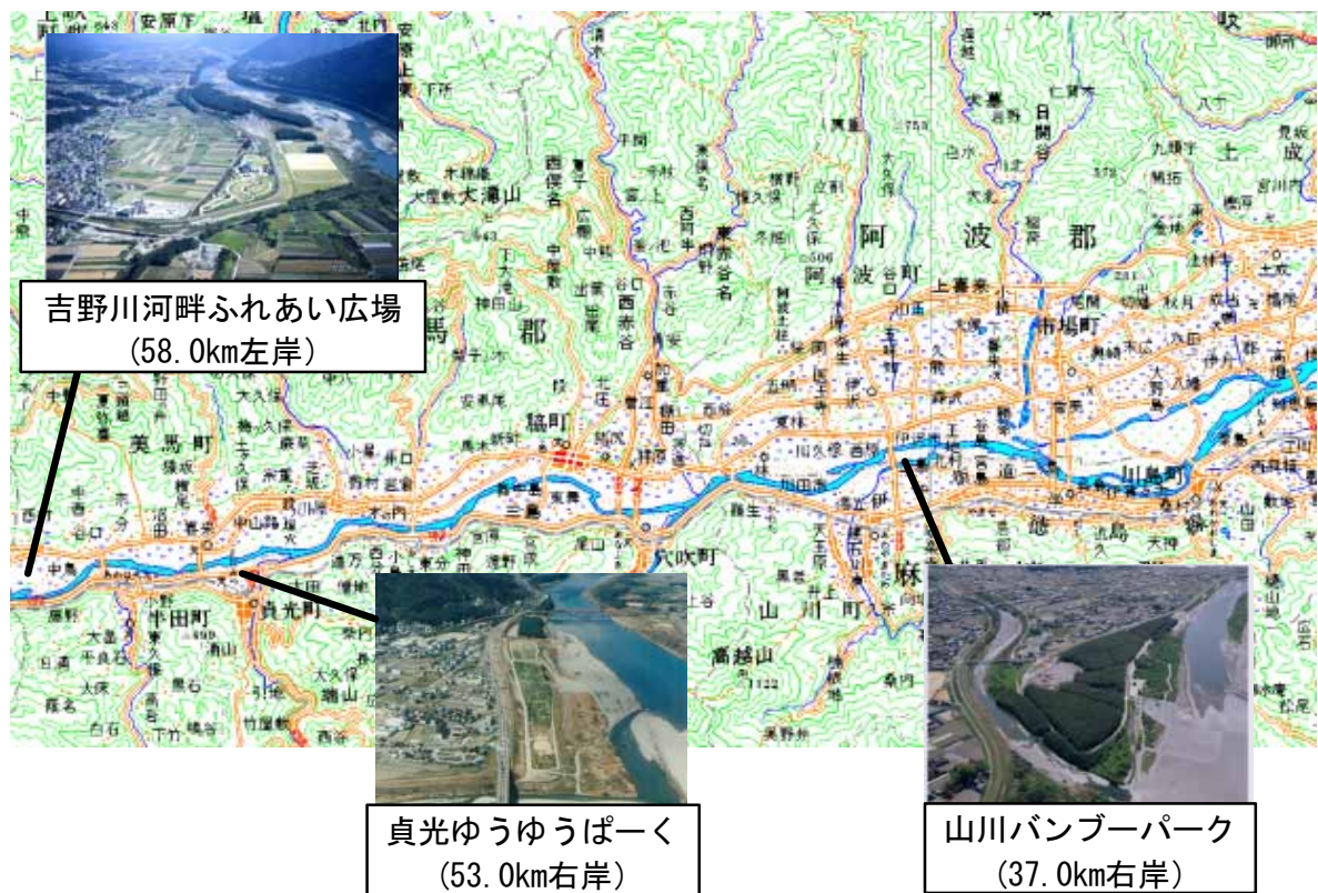
図-7.14(2) 吉野川(28.0k付近～58.0k付近)
