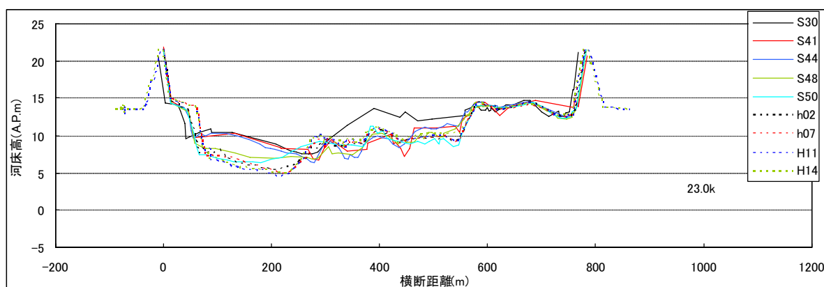
図－8. 2 (1) 横断形状の経年変化 (23. 0k)
