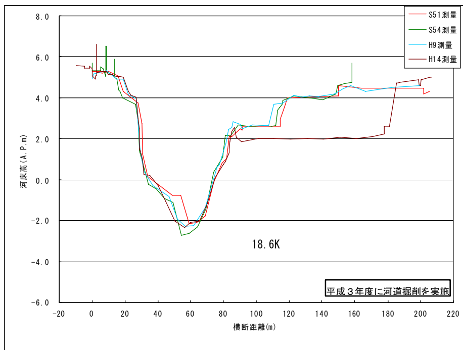
図8. 6(2) 横断形状の経年変化（大寺橋付近18. 6k）
