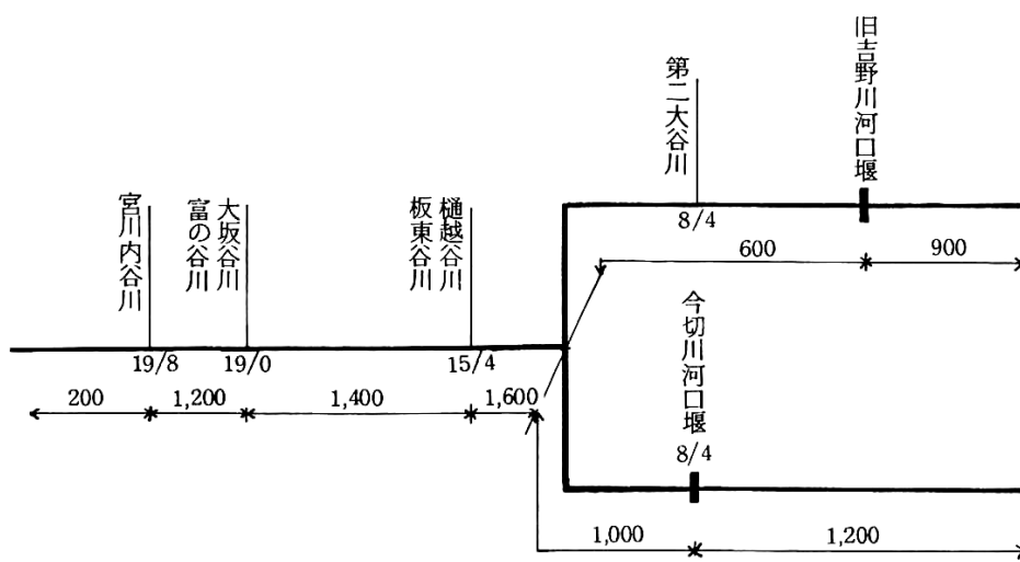
図-4. 16(2) S51.5改修計画(1/100規模)
