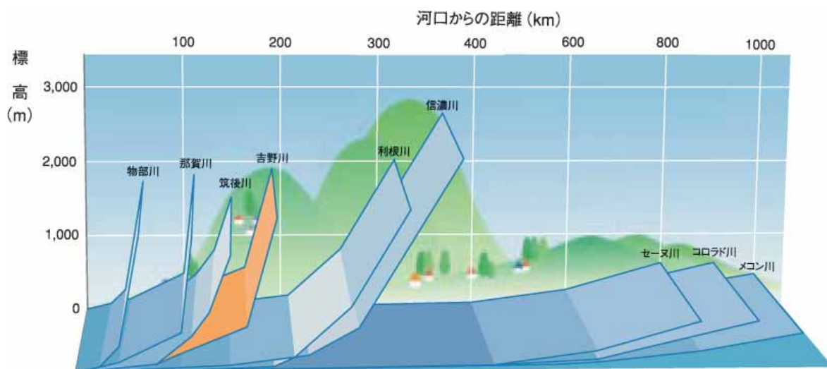
図－8.1 吉野川の河床勾配(他河川との比較)
