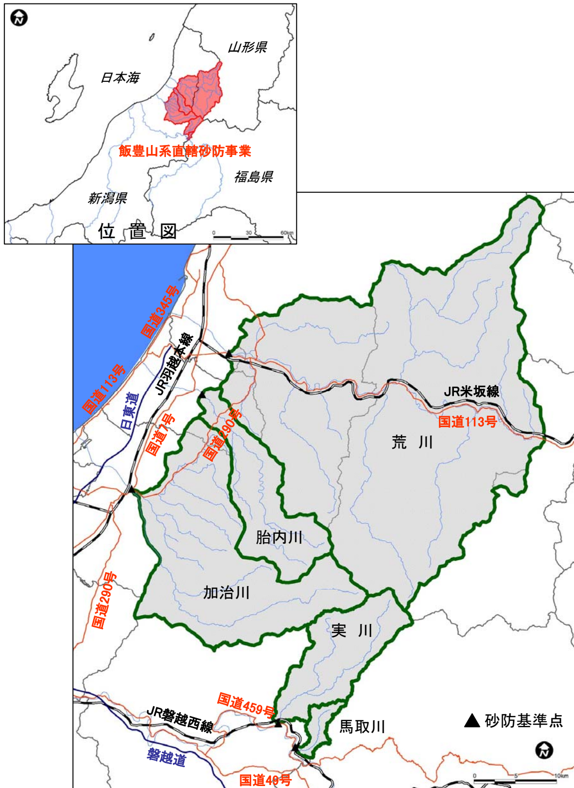
飯豊山系流域図
