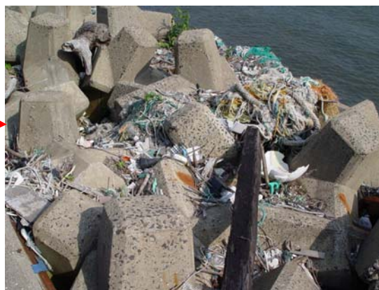
■ 消波機能が損なわれた消波工
