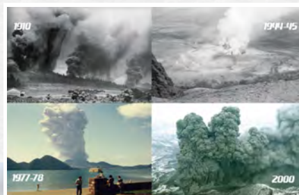
噴火を繰り返す有珠山(20世紀4回の噴火)
