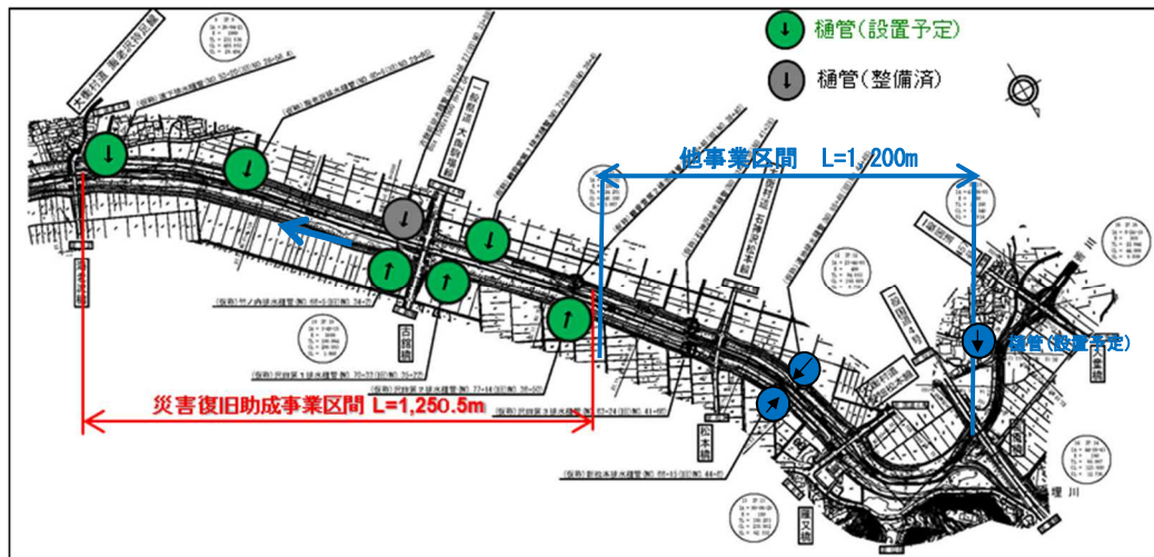
平面図
