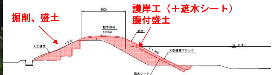
横断図（左岸）
