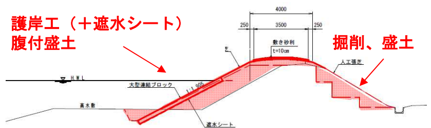
横断図（右岸）
