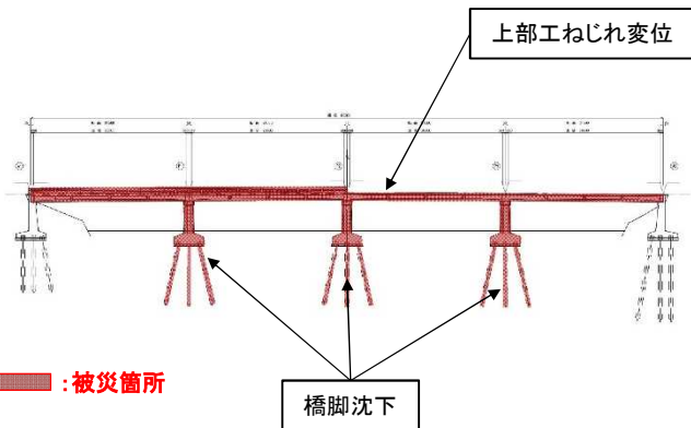
側面図
