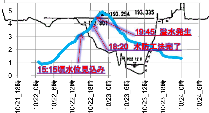
■ 現場付近の河川横断図と水位グラフ
