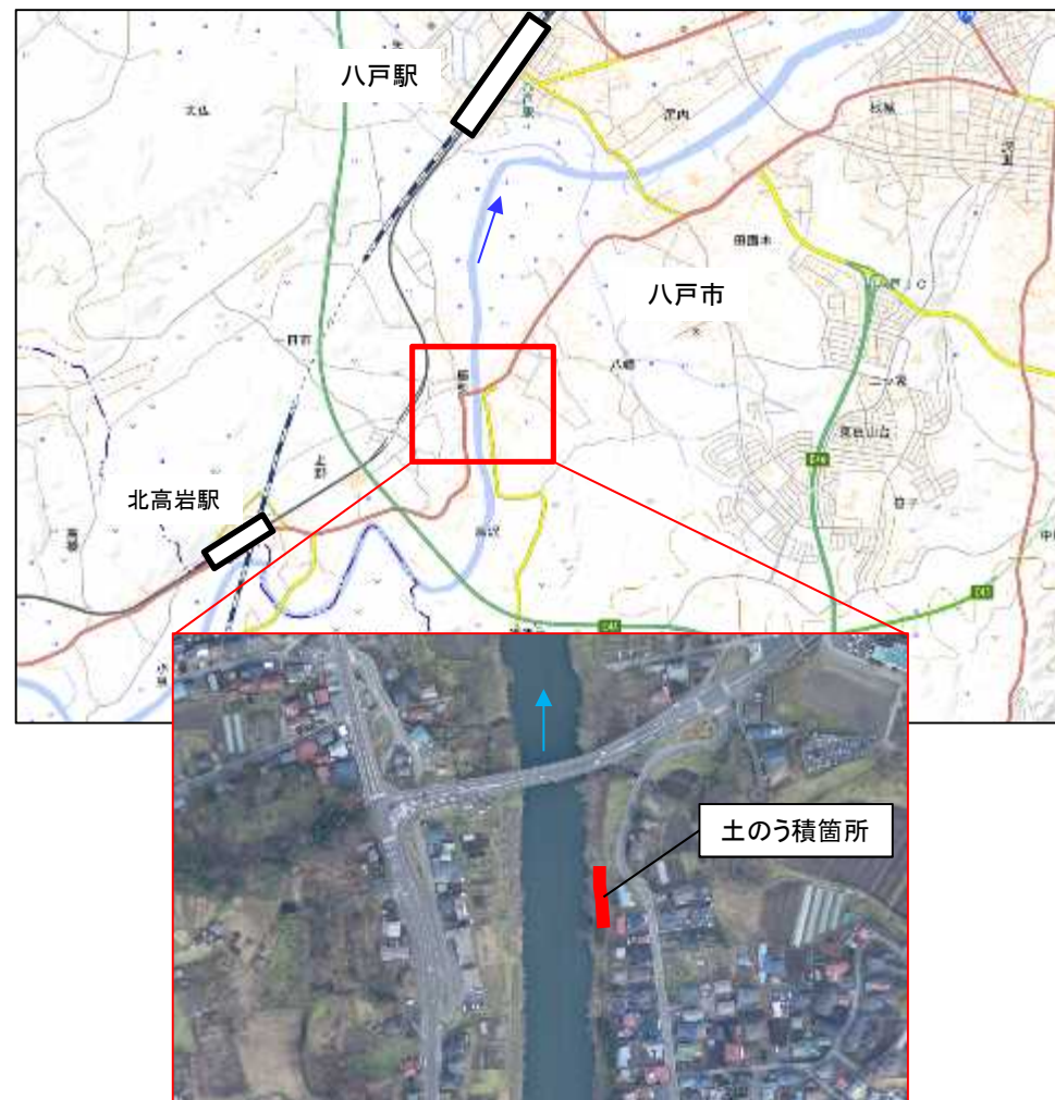
馬淵川右岸(八戸市櫛引地先) 積み土のう工
